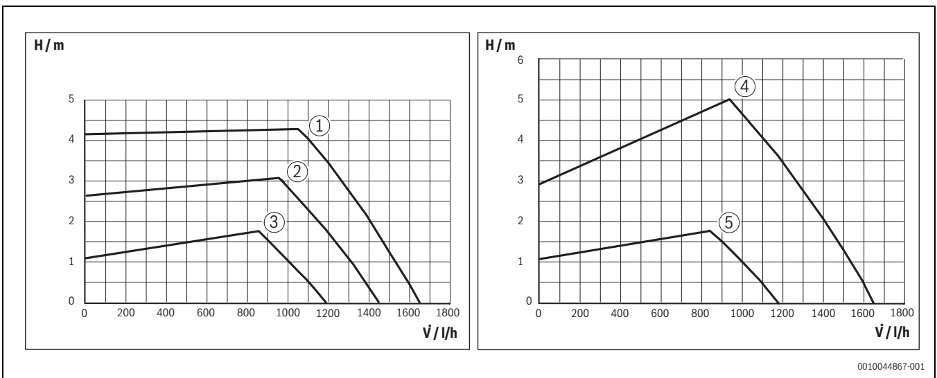
Bild 2 Pumpenkennfeld
