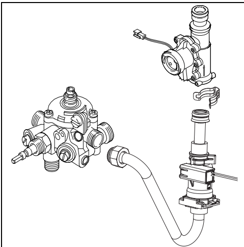
Bild 11 Einbau
