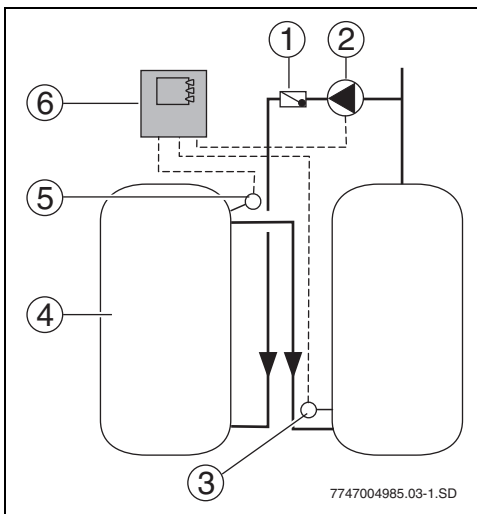
Bild 4 Umschichtfunktion
