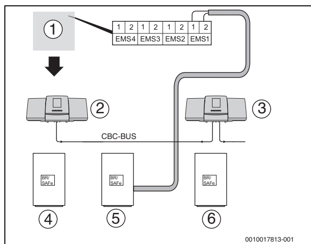
Bild 7 Mehrkesselanlage mit Logamatic 5000/Control 8000 und EMS-Regelung
