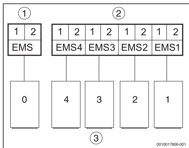
Bild 4 EMS-Anschlussklemmen
