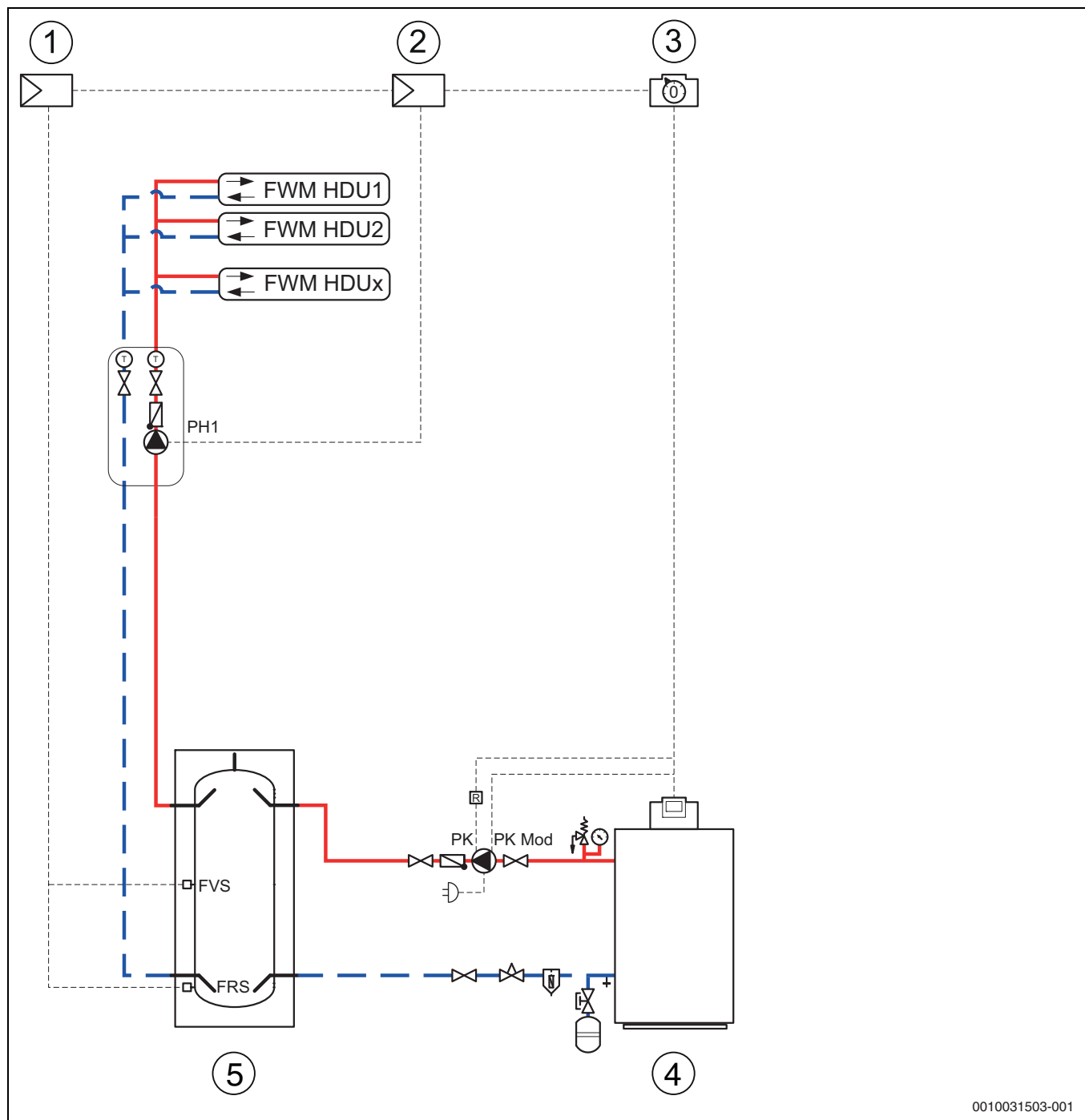
Bild 27 Wärmerezeuger mit Feuerungsautomat SAFe
