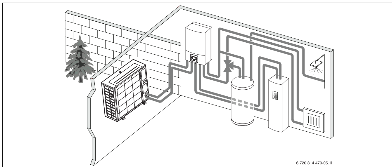
Bild 2 Wärmepumpe Außeneinheit, Inneneinheit ASB ohne elektrischen Zuheizer, externer Warmwasserspeicher und externer Zuheizer
