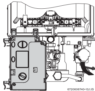
Fig. 2 Caixa de comando - posição de ajuste de gás
