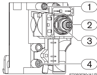
Bild 3 Druckmesspunkte
