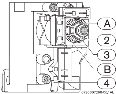
Fig. 4 2 Vis de réglage de débit gaz minimum 3 Ecrou de blocage du régulateur 4 Point de mesure de la pression du raccordement de gaz A Corps en laiton B Bague de blocage
