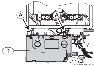
Fig. 1 Retirada de la caja de mando
