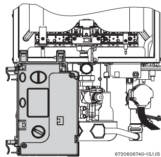
Fig. 2 Caja de mando - posición de ajuste del gas
