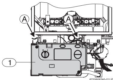
Rys. 1 Wyjmowanie skrzynki sterowniczej
