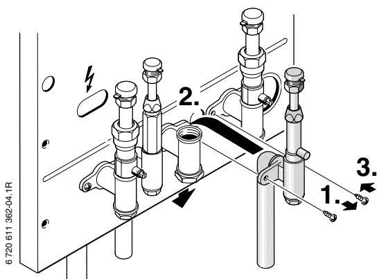
Bild 3 Kaltwasseranschluss montieren
