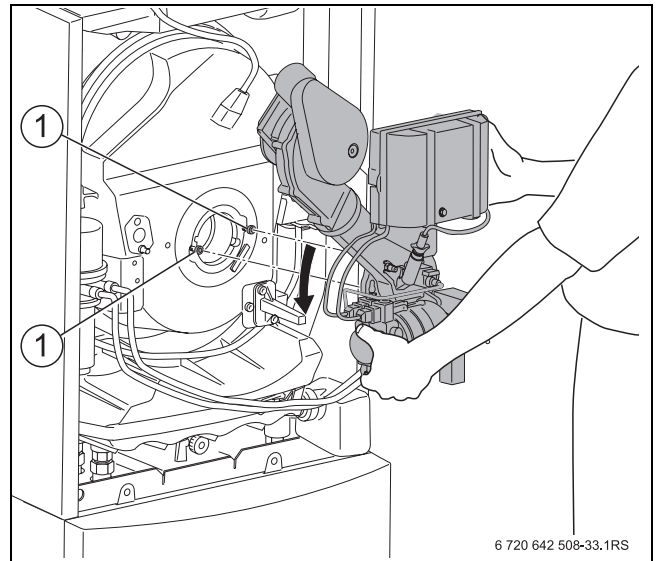
Bild 68 Brenner herausnehmen
