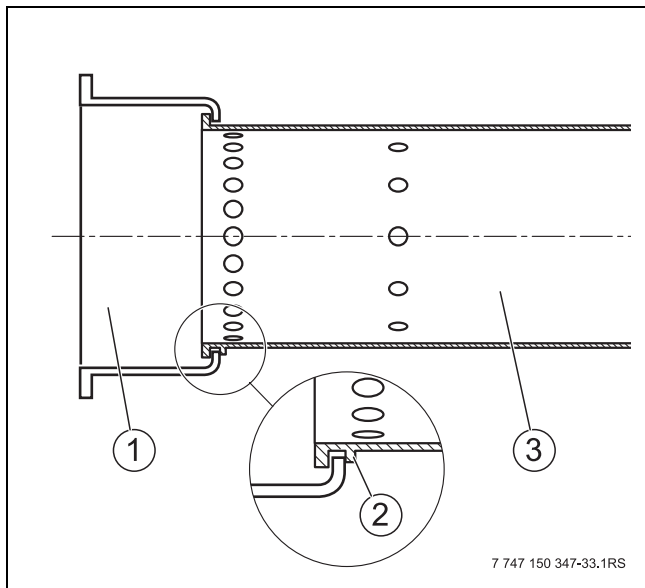
Bild 55 Brennerrohr einsetzen
