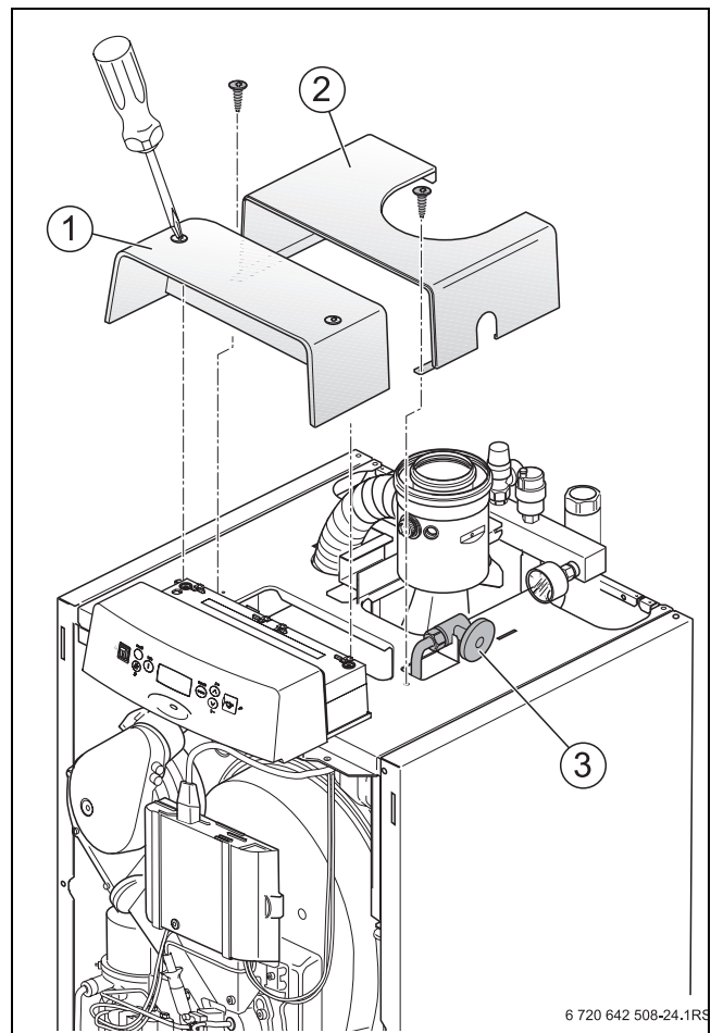
Bild 27 Ölleitung anschließen
