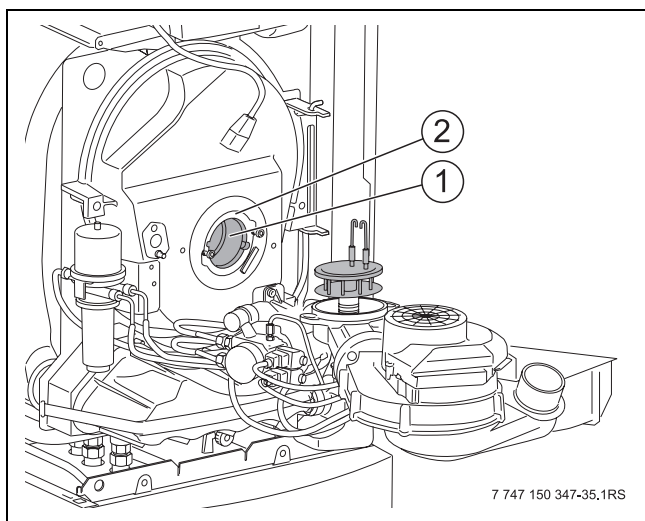
Bild 56 Dichtung prüfen
