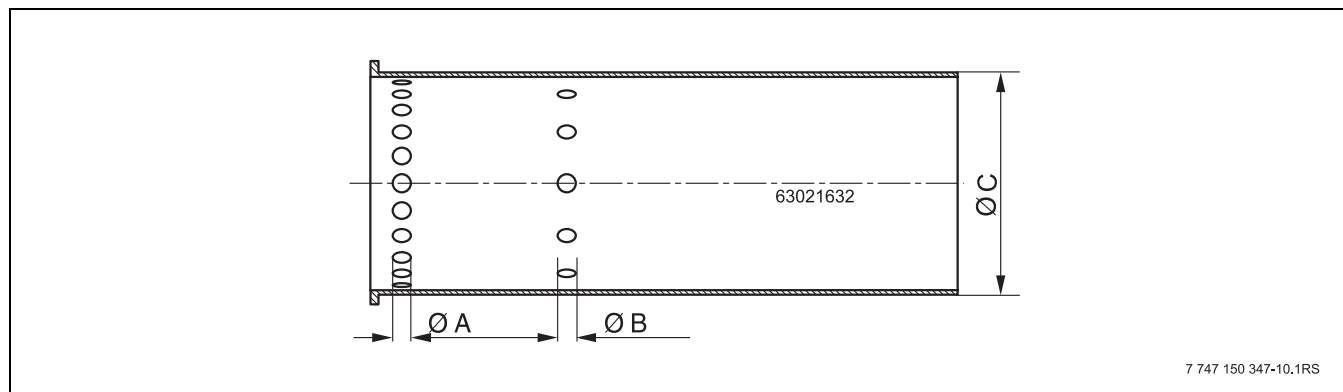
Bild 7 Brennerrohre
