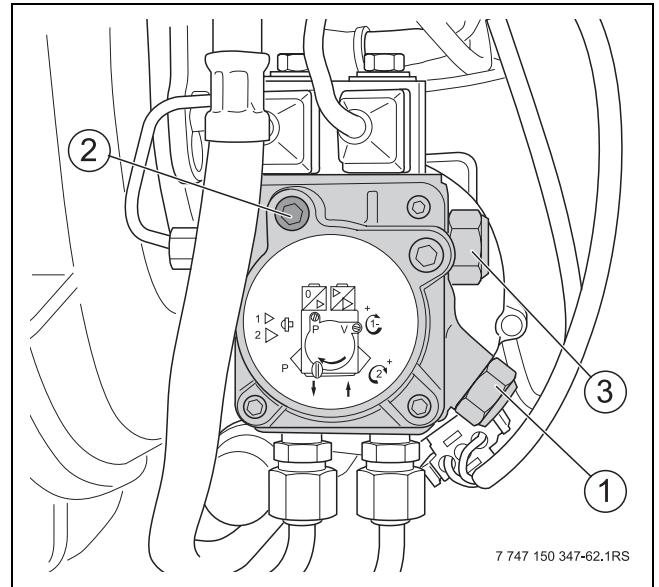
Bild 40 Druck einstellen
