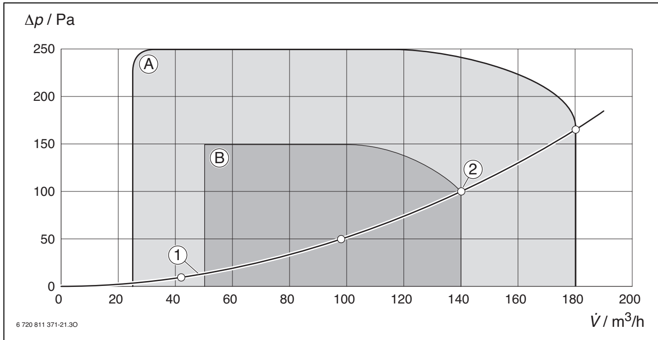
Bild 62 Kennlinien Druckerhöhung/Volumenstrom HR 140 W(S)
