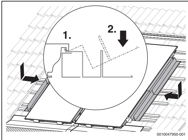
Bild 59 Seitliche Eindeckbleche montieren
