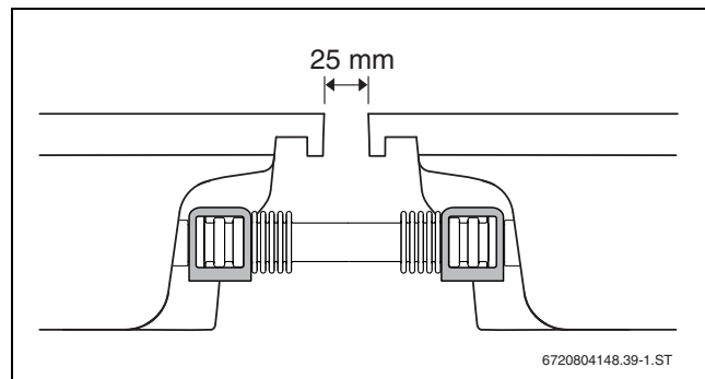
Bild 46 Hydraulische Verbindung zweier Kollektoren
