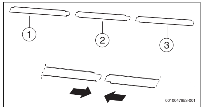
Bild 62 Unterschiedliche Formen von Blenden (hier: Typ senkrecht für 3 Kollektoren)
