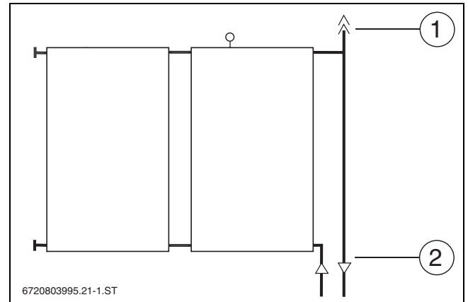
Bild 54 Hydraulischer Anschluss mit Entlüfter (Vorlauf rechts)
