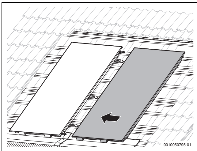
Bild 44 Rechten Kollektor nach links schieben
