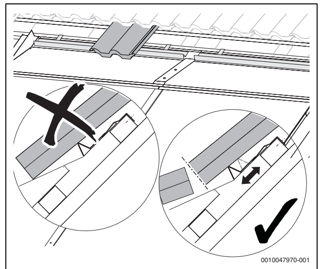
Bild 78 Dachziegelaufgabe positionieren
