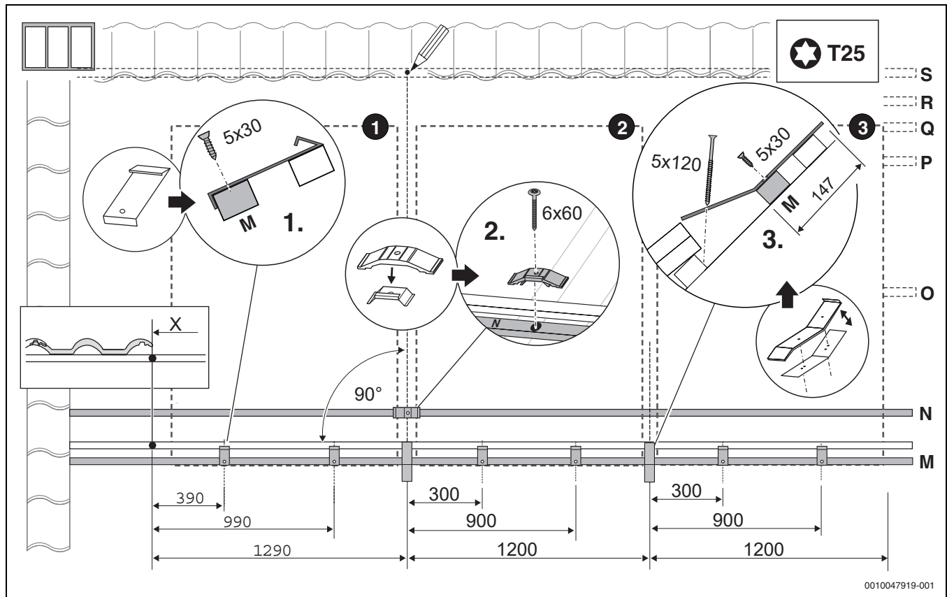
Bild 27 Kollektortyp senkrecht (3 Kollektoren), Maße in mm
