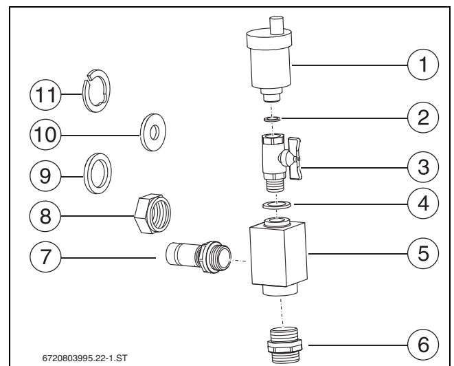
Bild 55 Lieferumfang Entlüfter-Set
