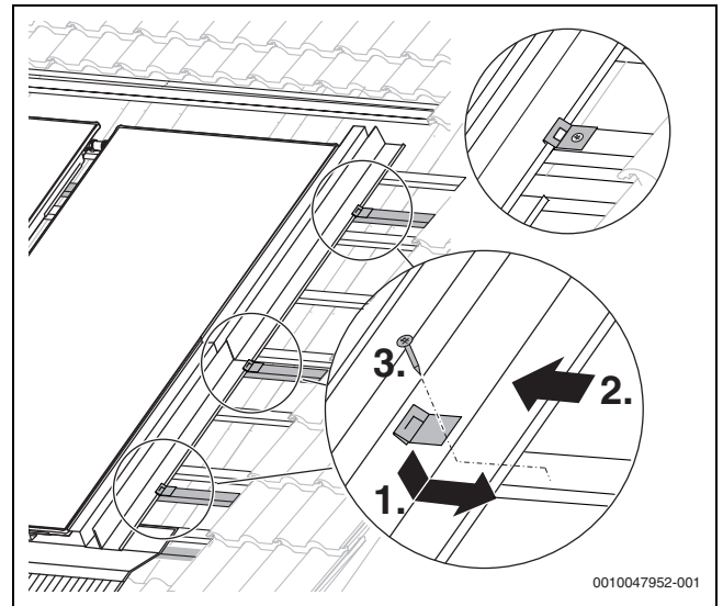
Bild 61 Hafter montieren
