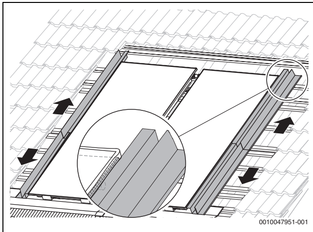
Bild 60 Seitliche Eindeckbleche auseinanderziehen (senkrecht)
