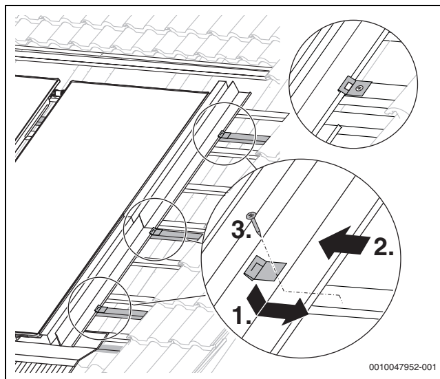
Bild 65 Hafter montieren
