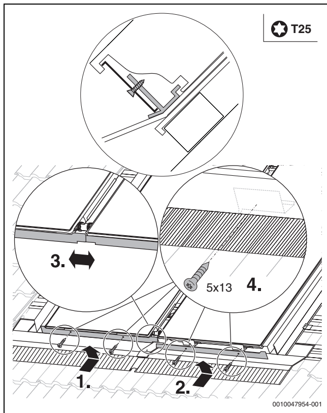
Bild 67 Blenden festschrauben
