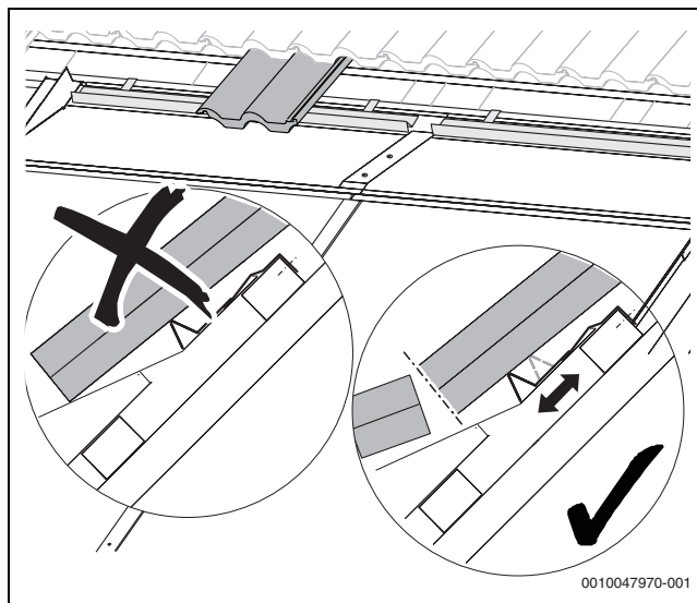
Bild 82 Dachziegelaufgabe positionieren
