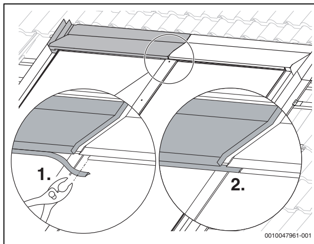
Bild 74 Dichtlippe anpassen
