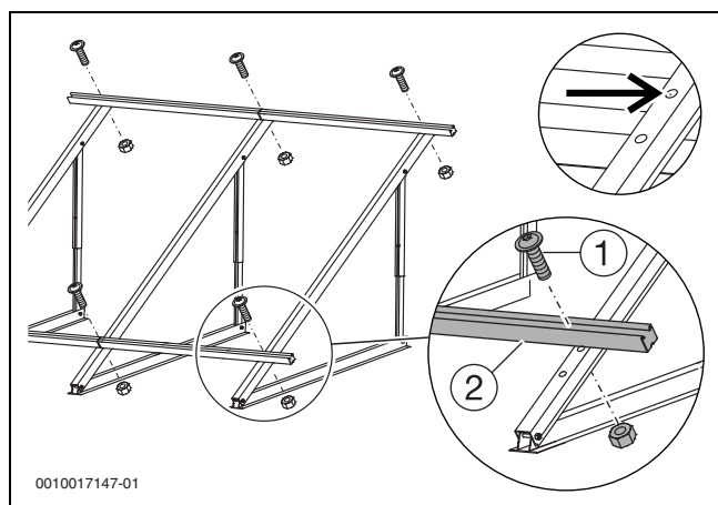
Bild 30 Profilschienen montieren
