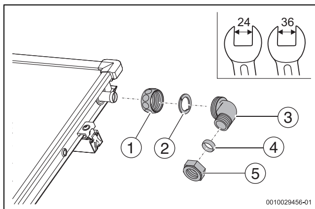
Bild 51 Winkeltülle montieren
