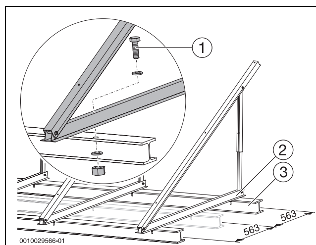
Bild 25 Kollektorstützen auf Doppel-T-Träger, Maße in mm
