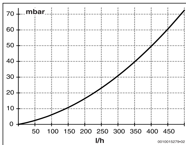
Bild 2 Druckverlustkurve (Wasser-Glykol-Gemisch)
