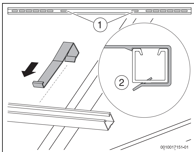
Bild 33 Abrutschsicherung an Profilschiene unten montieren
