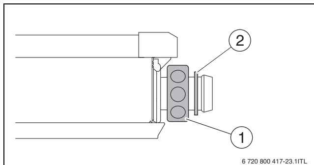
Bild 50 Anschluss der Rohrleitung vorbereiten
