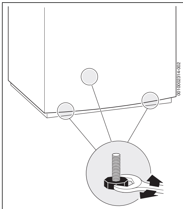
Bild 46 Speicher ausrichten
