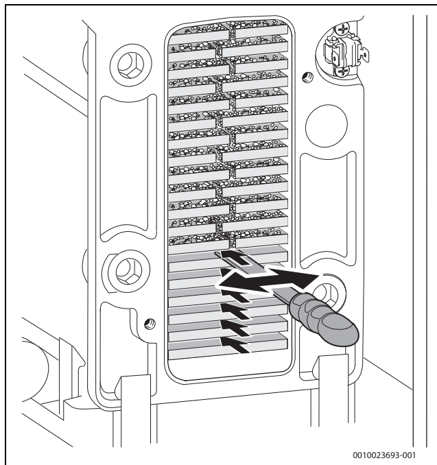
Bild 209 Reinigungsmesser
