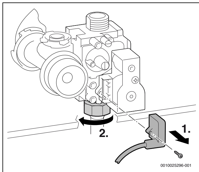
Bild 220 Stecker abziehen und Überwurfmutter lösen
