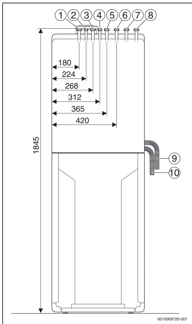
Bild 5 Anschlussmaße des Zubehörs CS 11 - Vertikales Anschluss-Set (Maße in mm)
