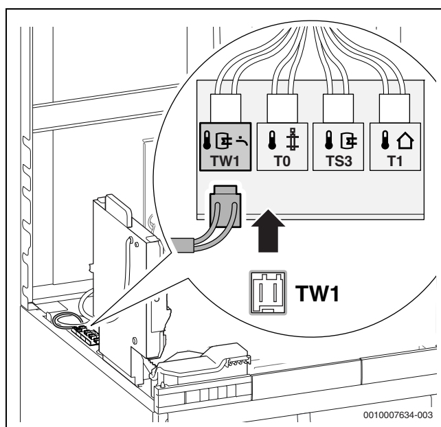
Bild 59 Speichertemperaturfühler anschließen
