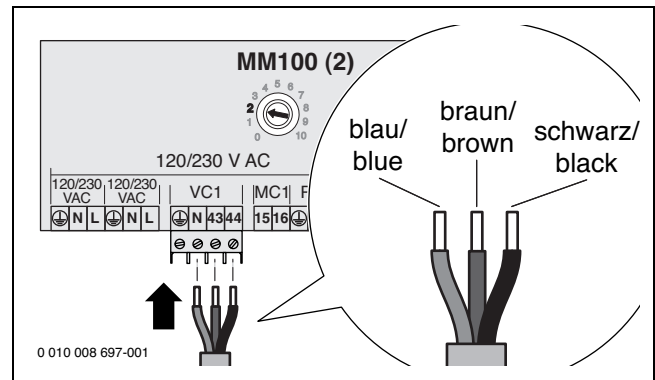
Bild 140 Anschluss Kabel Mischermotor am Modul MM 100 [2]
