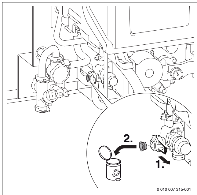
Bild 113 Stopfen entfernen
