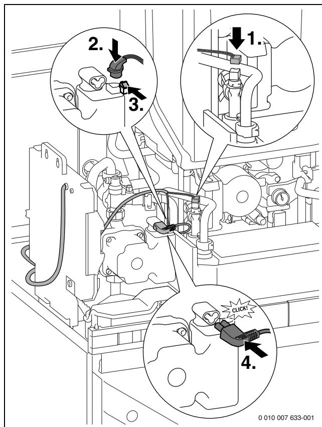
Bild 58 Speicherladepumpe und Warmwasser-Temperaturfühler anschließen
