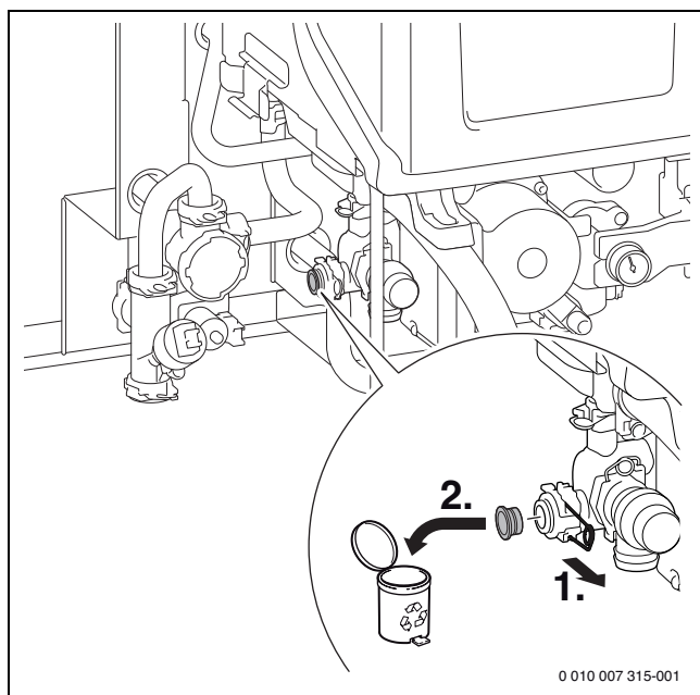
Bild 142 Stopfen entfernen
