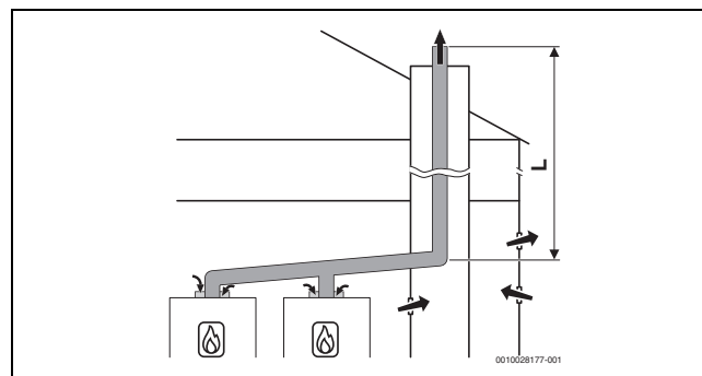
Bild 36 Kaskade mit 2 Geräten: Starre Abgasführung im Schacht nach B 23p /B 53p mit raumluftabhängiger Luftzufuhr am Gerät
