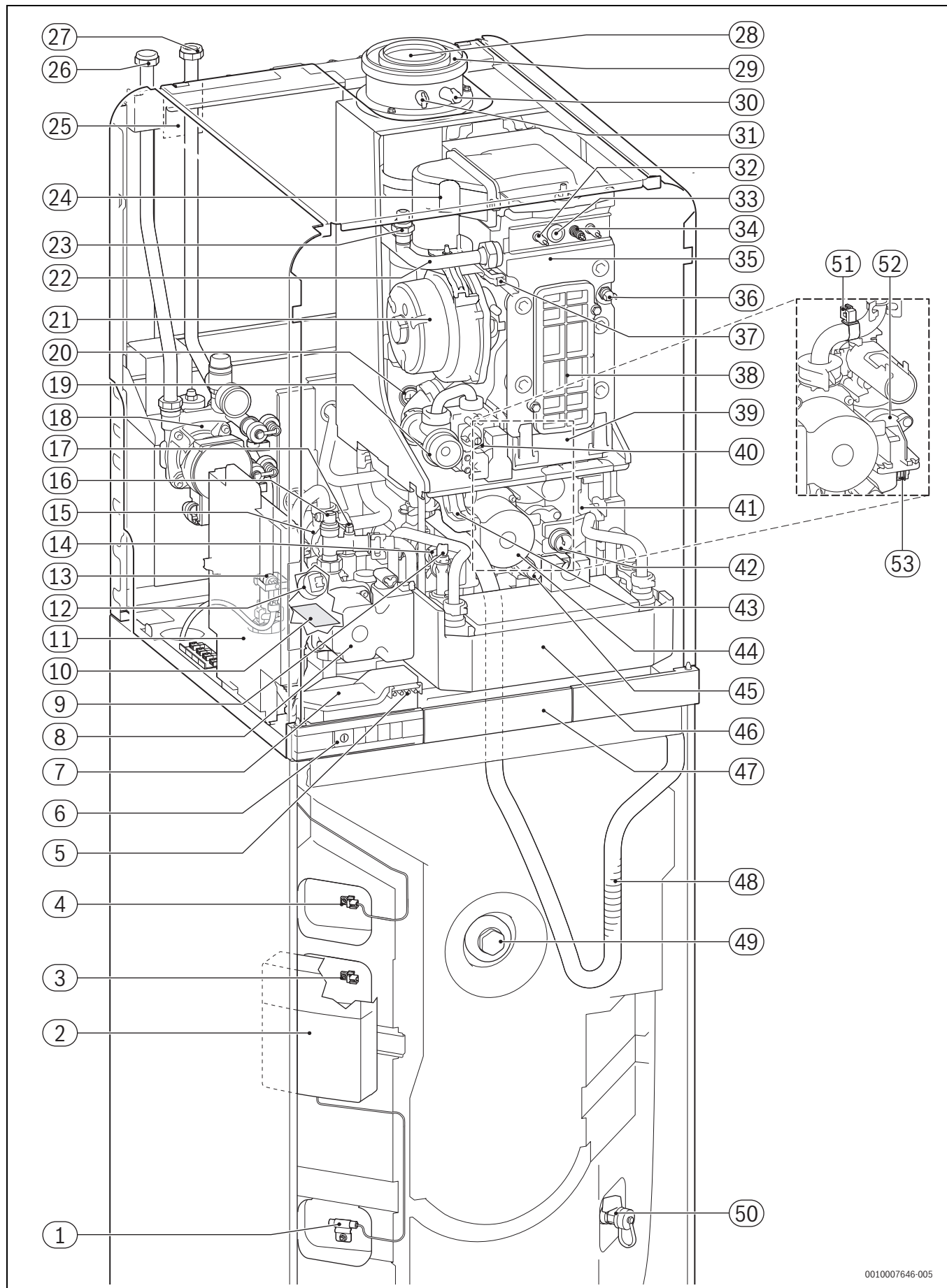
Bild 12 GC9000iWM.../210 S-Geräte
