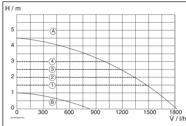
Bild 227 Pumpenkennfelder und Pumpenkennlinien
