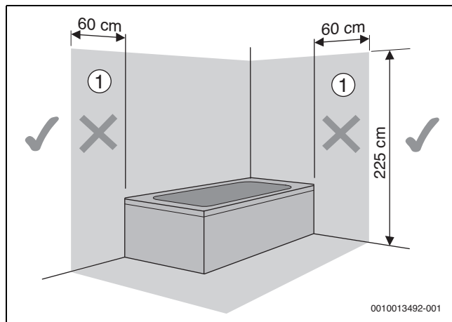
Bild 176 Schutzbereiche
