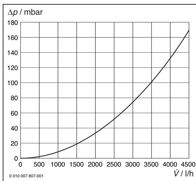
Bild 230 Druckverlust-Diagramm gemischter Heizkreis (HK2)
