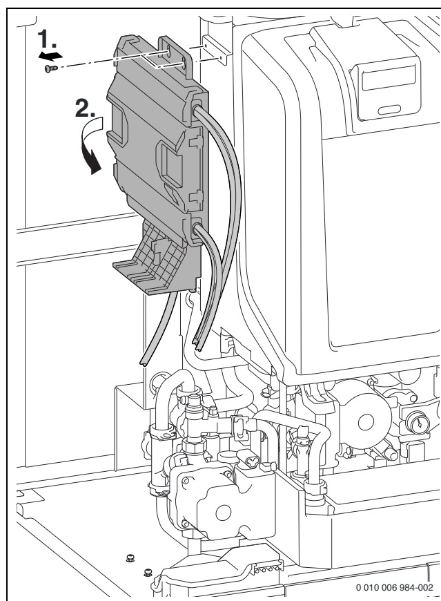
Bild 55 Steuergerät abnehmen
