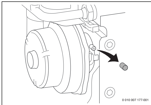
Bild 208 Messstutzen an der Mischeinrichtung
