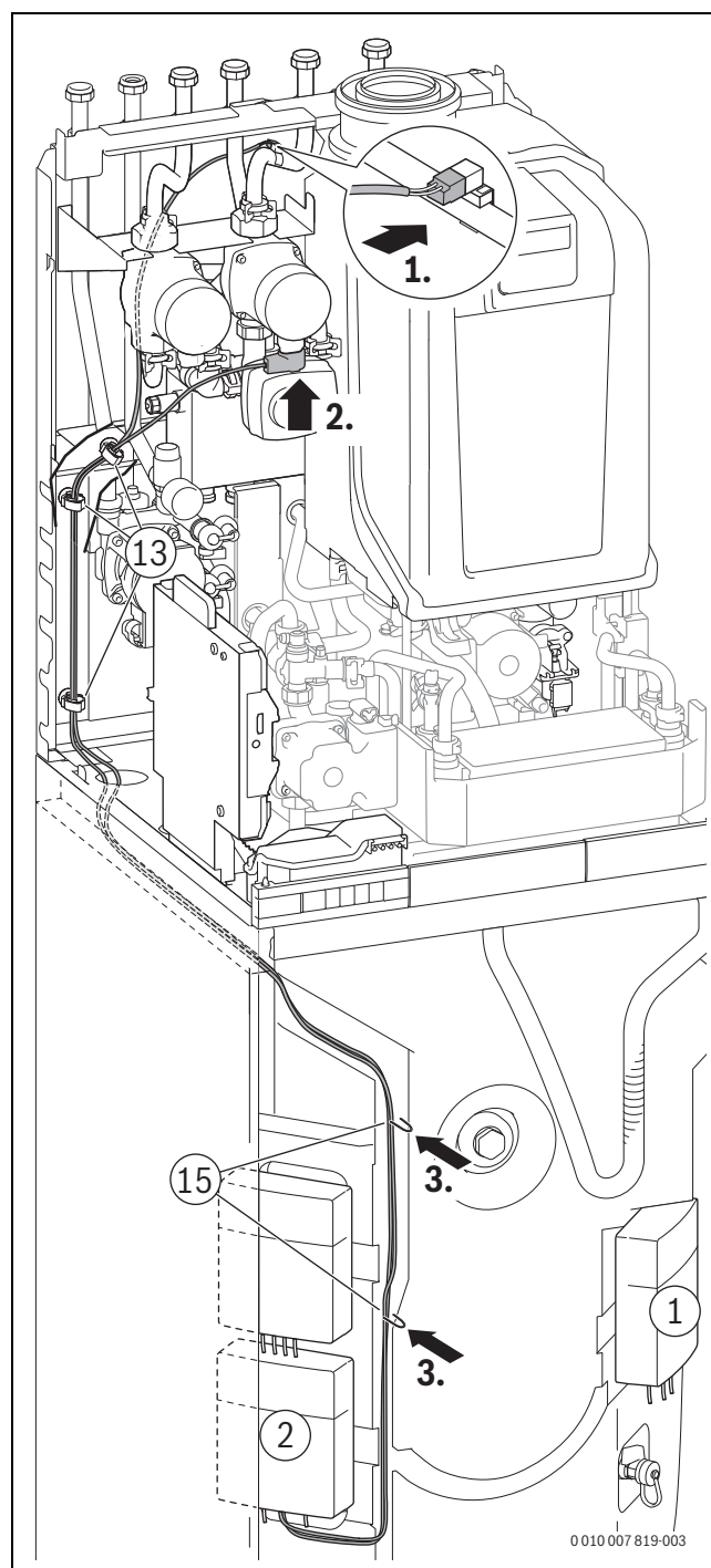
Bild 137 Anschluss Heizungspumpe gemischter Heizkreis und Temperaturfühler
