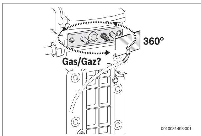
Bild 205 Dichtheit kontrollieren
