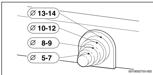
Bild 139 Zugentlastung Kabel Mischermotor anpassen
