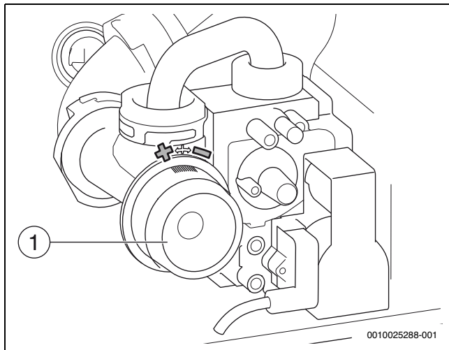
Bild 199 Gas-Luft-Verhältnis einstellen
