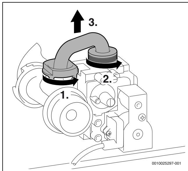
Bild 219 Gasrohr ausbauen
