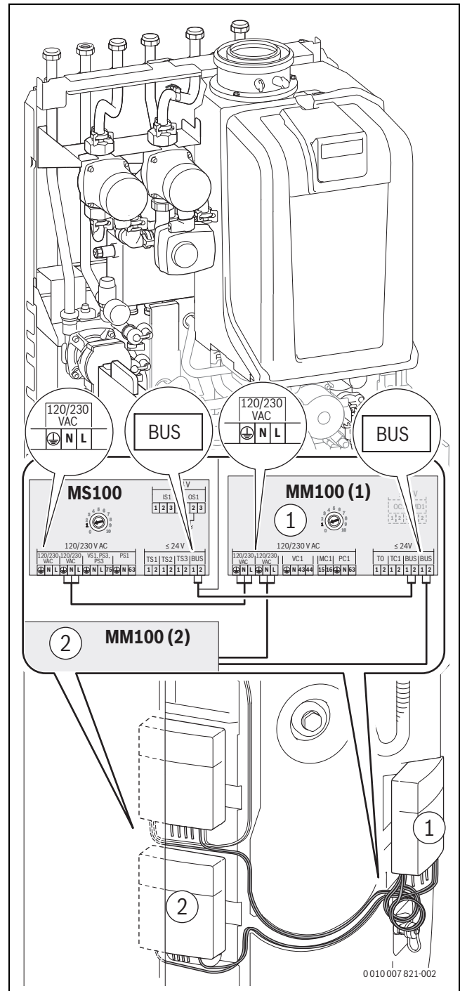
Bild 141 Anschluss am Modul MS 100 und am Modul MM 100 durchschleifen
