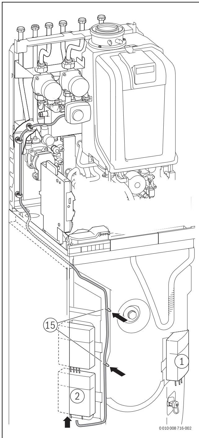
Bild 138 Anschluss Mischermotor
