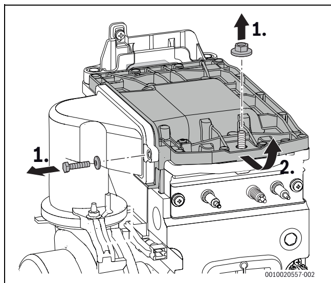
Bild 206 Brennerdeckel ausbauen
