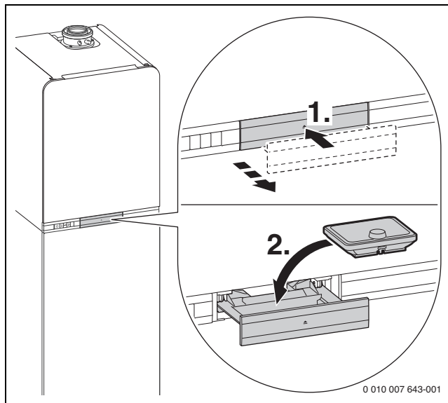
Bild 184 Heizungsregler einstecken
