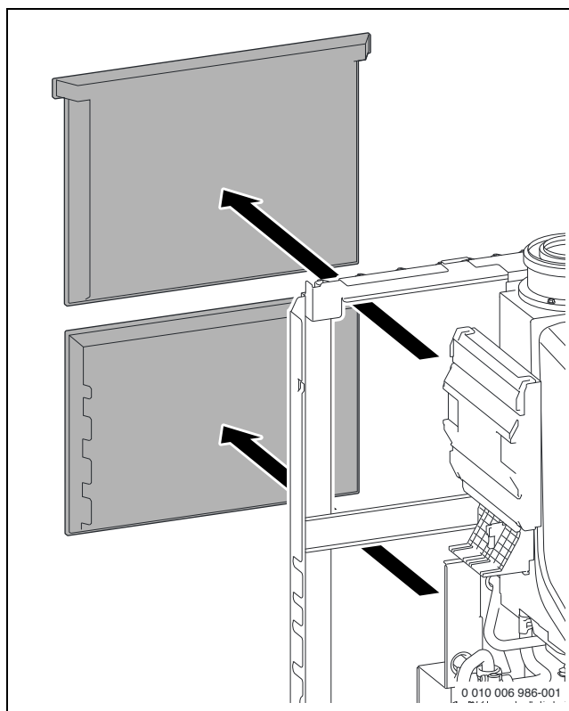
Bild 64 Wärmedämmungen an der Rückseite abnehmen
