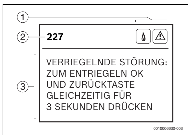
Bild 223 Störungsanzeige
