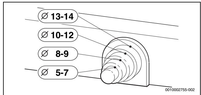
Bild 178 Zugentlastung an Kabeldurchmesser anpassen
