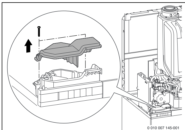
Bild 60 Abdeckung der Anschlussbox entfernen
