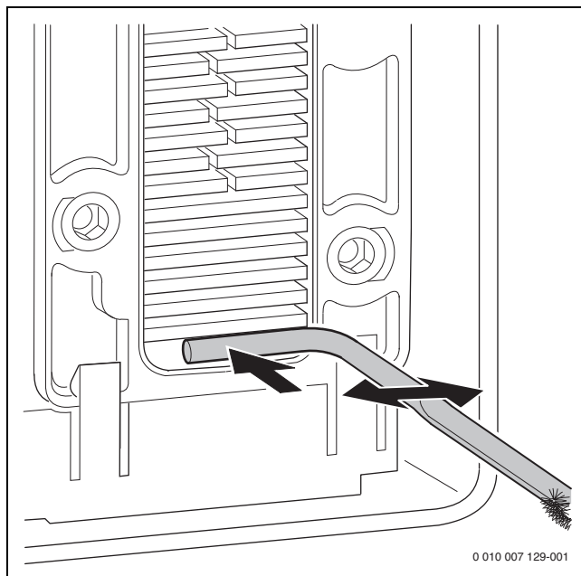
Bild 212 Kondensatwanne reinigen
