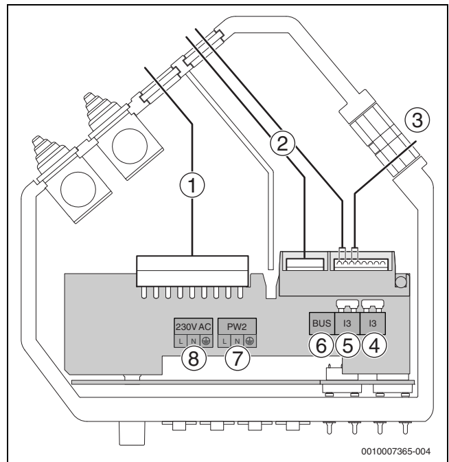
Bild 179 Anschlussbox
