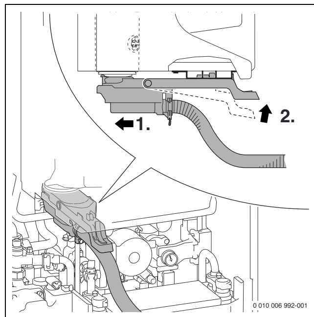
Bild 50 Schmutzfänger montieren
