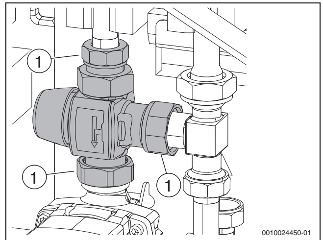
Bild 38 3-Wege-Ventil
