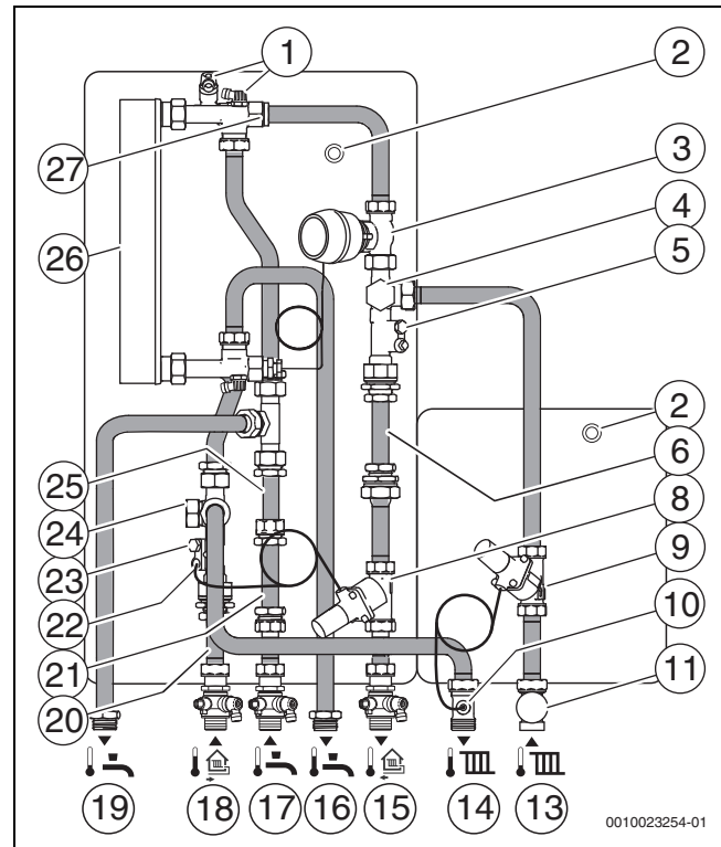
Bild 3 Station mit Modul ungemischter Heizkreis und zusätzlichem Differenzdruckregler
