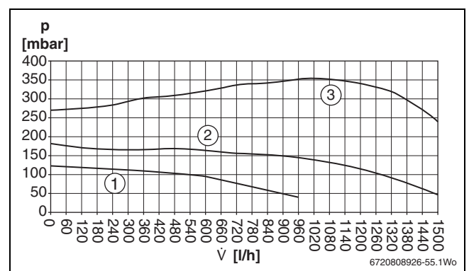
Bild 28 Restförderhöhe
