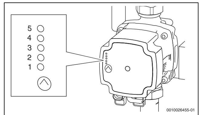
Bild 39 Störungsanzeigen der integrierten Heizungspumpe
