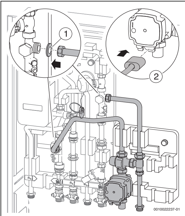
Bild 16 Heizkreismodul montieren
