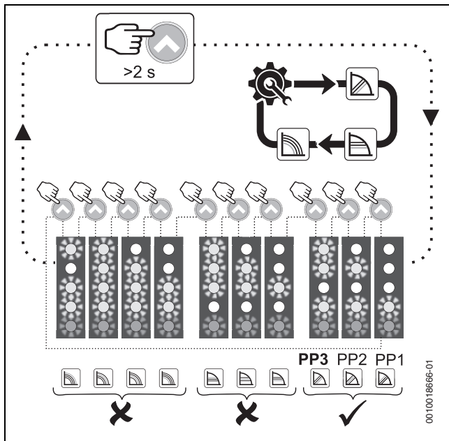
Bild 29 Einstellung der Pumpenkennlinie
