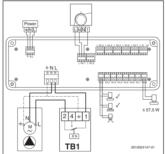
Bild 17 Elektrischer Anschluss an die Klemmleiste Fußbodenheizung (Zubehör)
