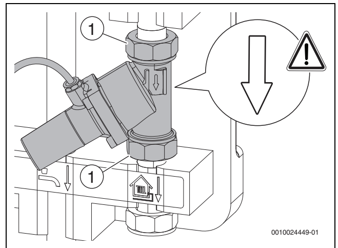
Bild 37 Differenzdruckregler
