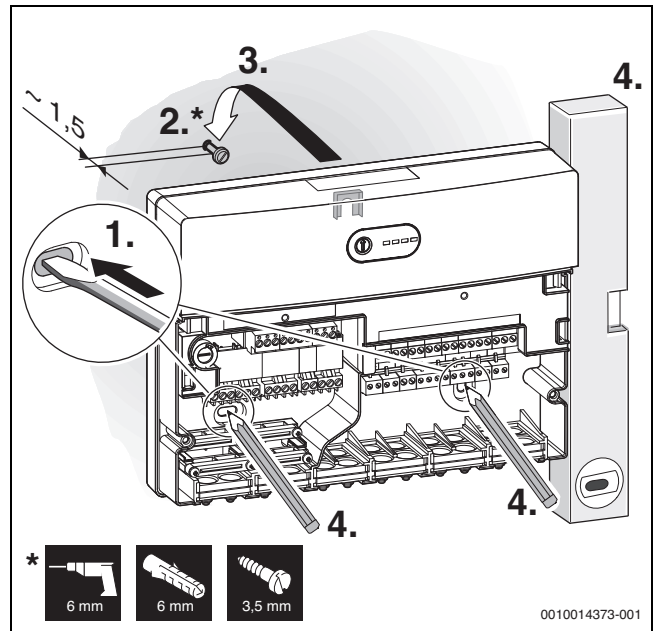
Bild 21 Wandbefestigung anzeichnen
