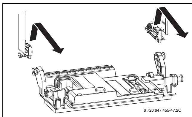
Bild 79 Steuergerät aushängen
