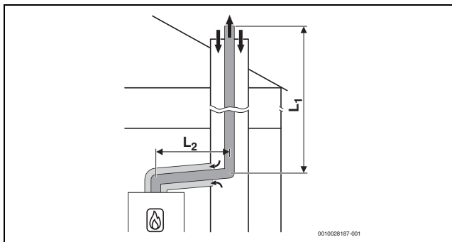
Bild 15 Starre Abgasführung nach C 93x im Schacht und konzentrische Luft-Abgas-Führung im Aufstellraum
