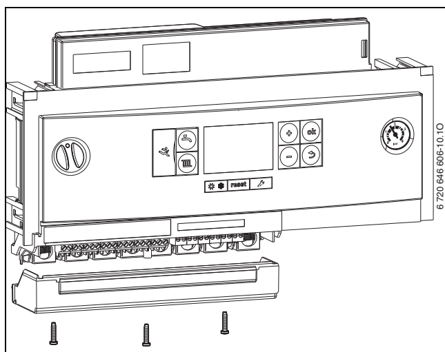
Bild 76 Abdeckung entfernen
