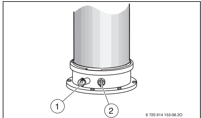
Bild 55 Abgassensstutzen und Verbrennungsluft-Messstutzen
