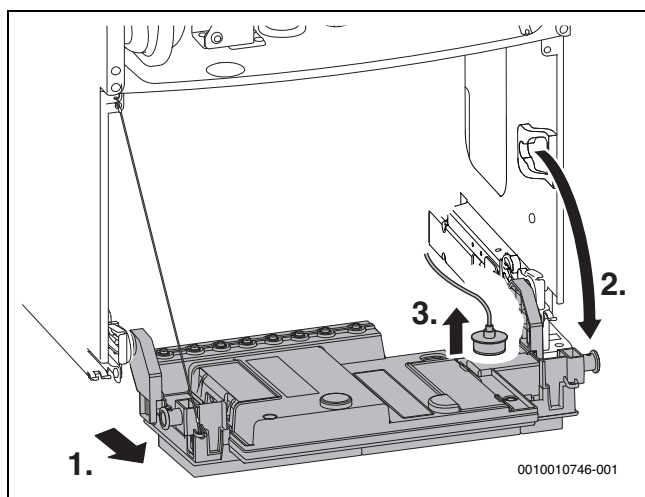
Bild 77 Steuergerät nach unten klappen
