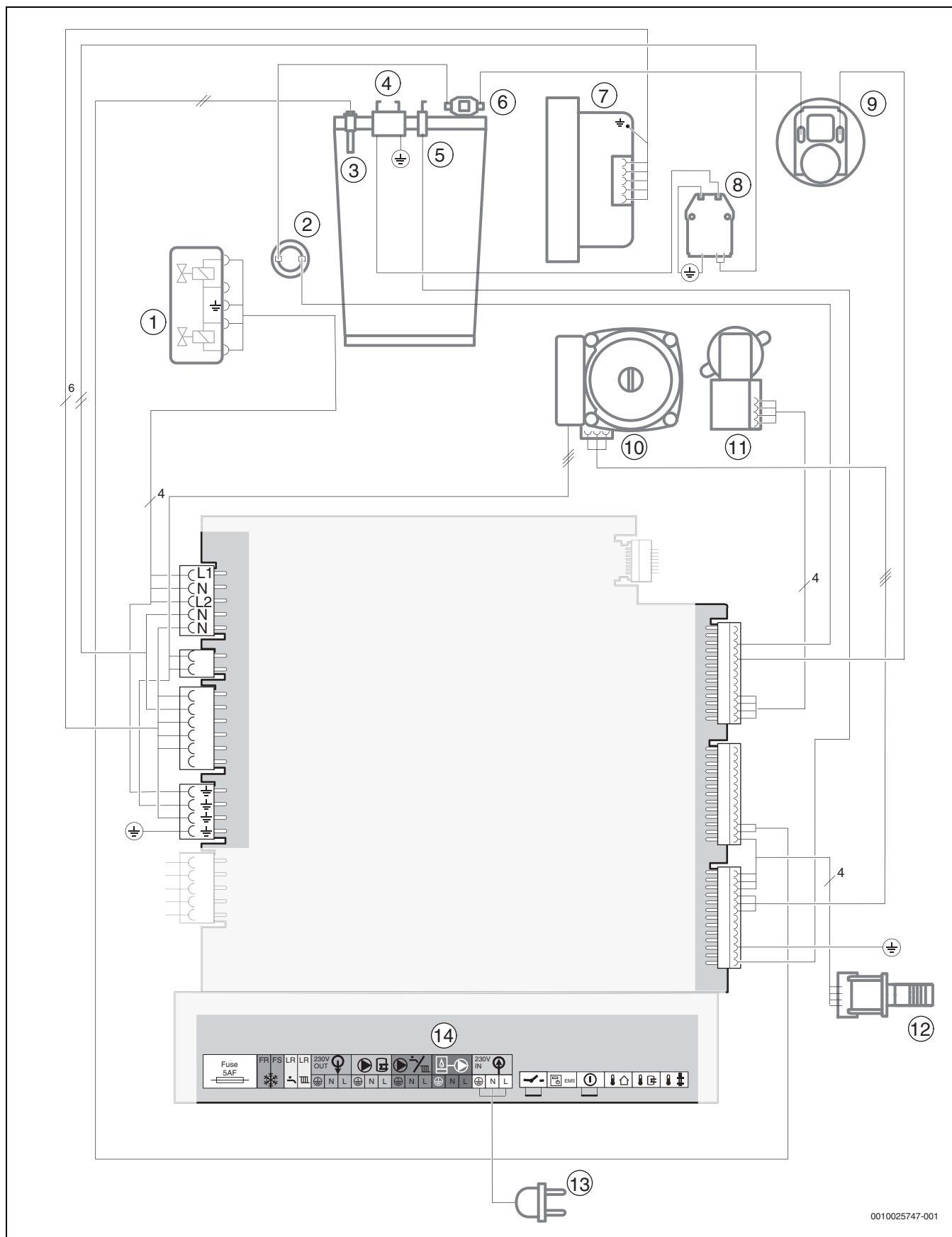
Bild 85 Elektrische Verdrahtung
