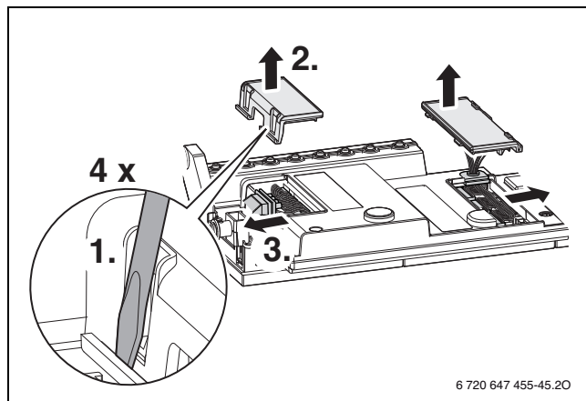
Bild 78 Abdeckung entfernen
