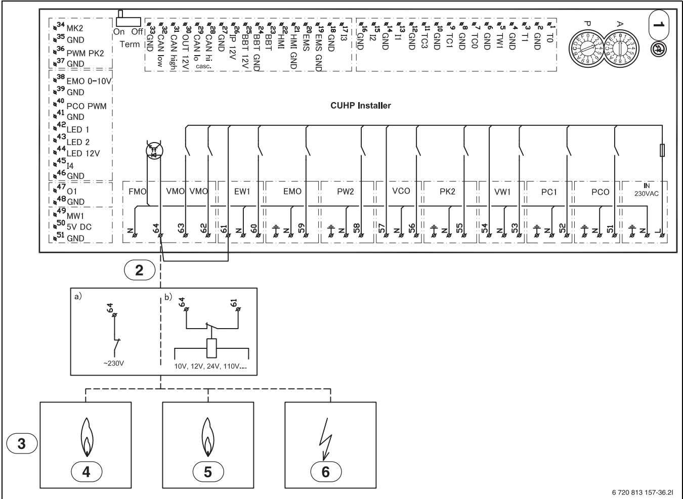
Bild 14 Schaltschema des Installationsmoduls, Alarm für externen Zuheizer
