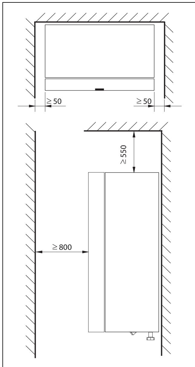
Bild 3 Mindestabstand (mm)
