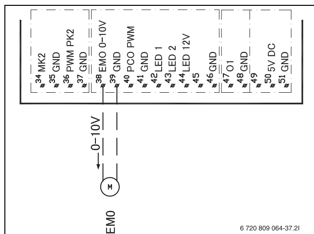
Bild 16 0- bis 10-V-Ansteuerung für externe Zuheizer
