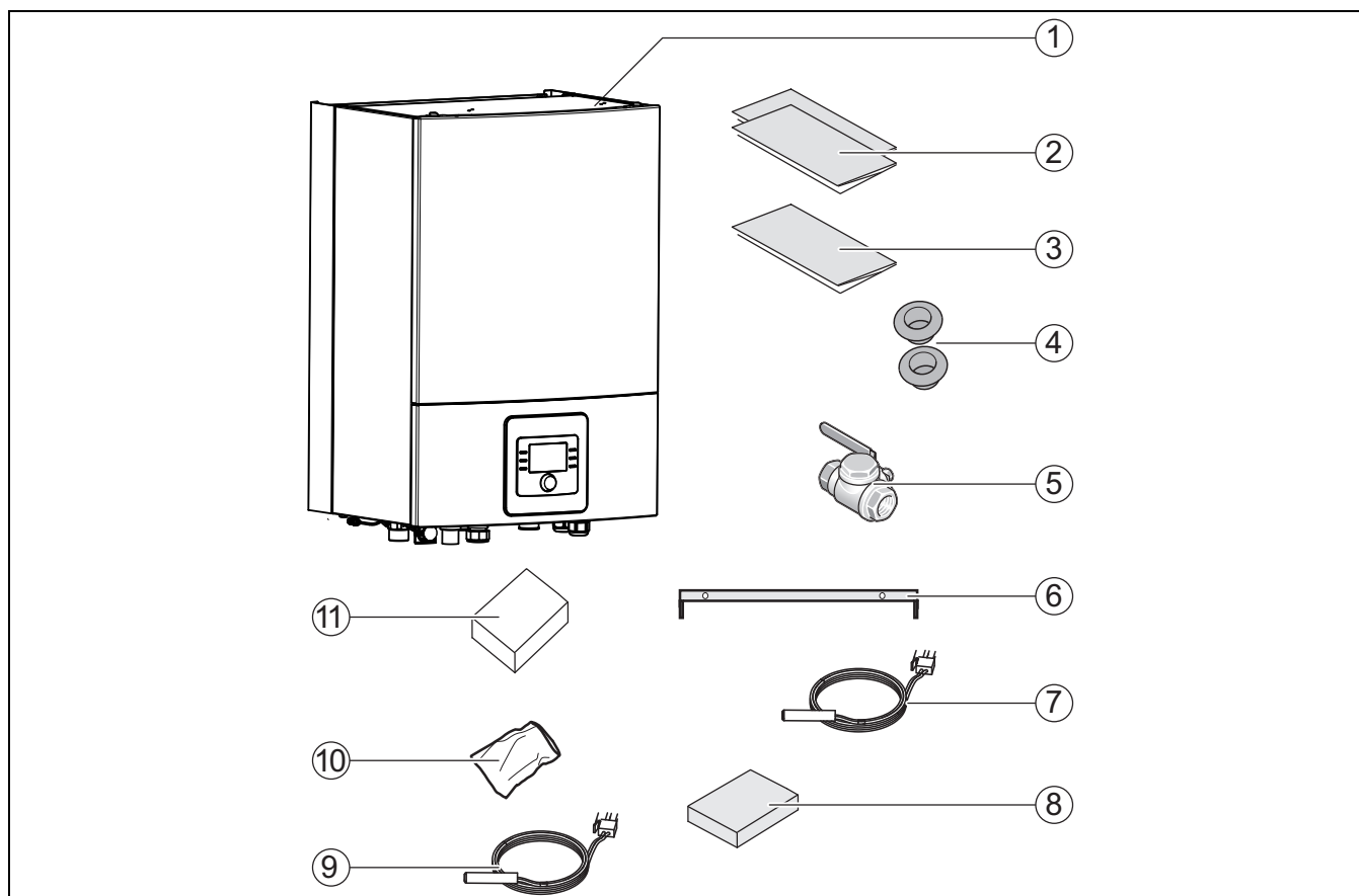
Bild 1 Lieferumfang
