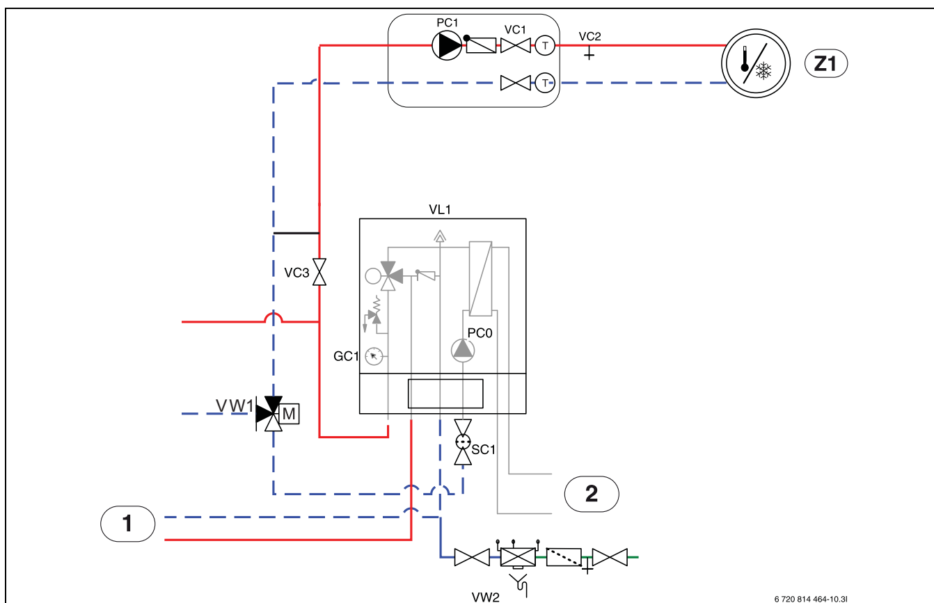
Bild 8 Inneneinheit mit externem Zuheizter und Heizsystem
