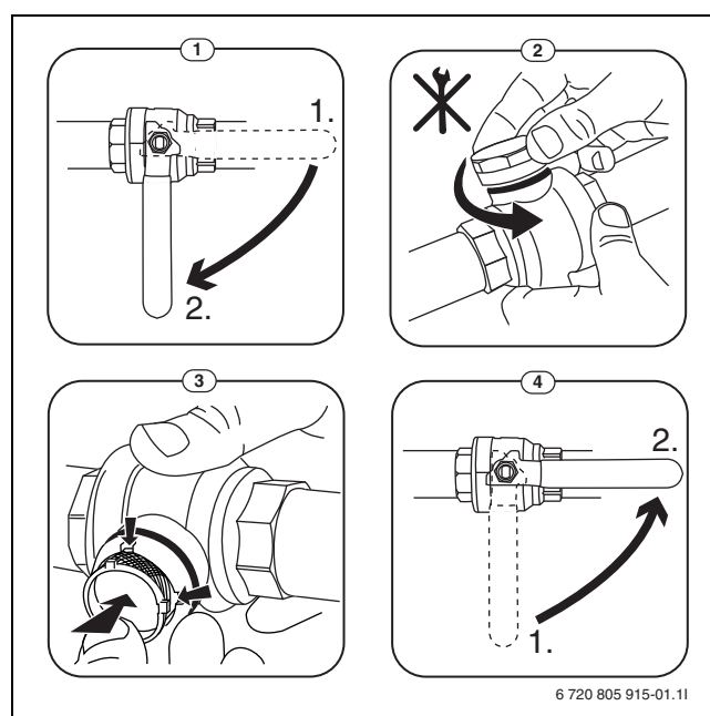
Bild 18 Siebreinigung
