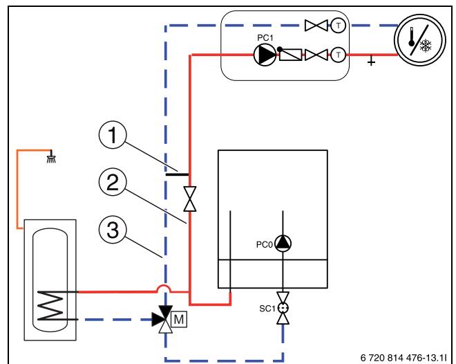
Bild 28 Inneneinheit mit Heizkreis und Warmwasserbereitung
