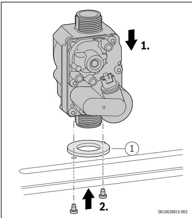
Bild 80 Gasarmatur einbauen
