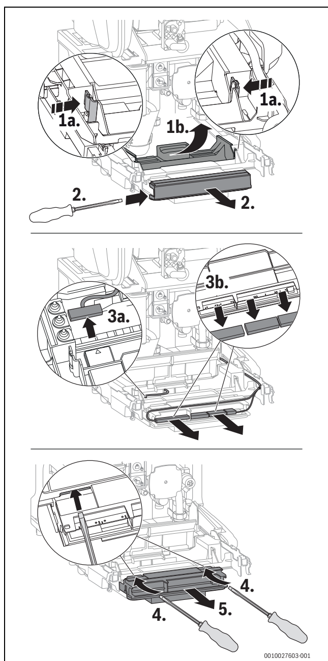
Bild 84 Steuergerät herausnehmen
