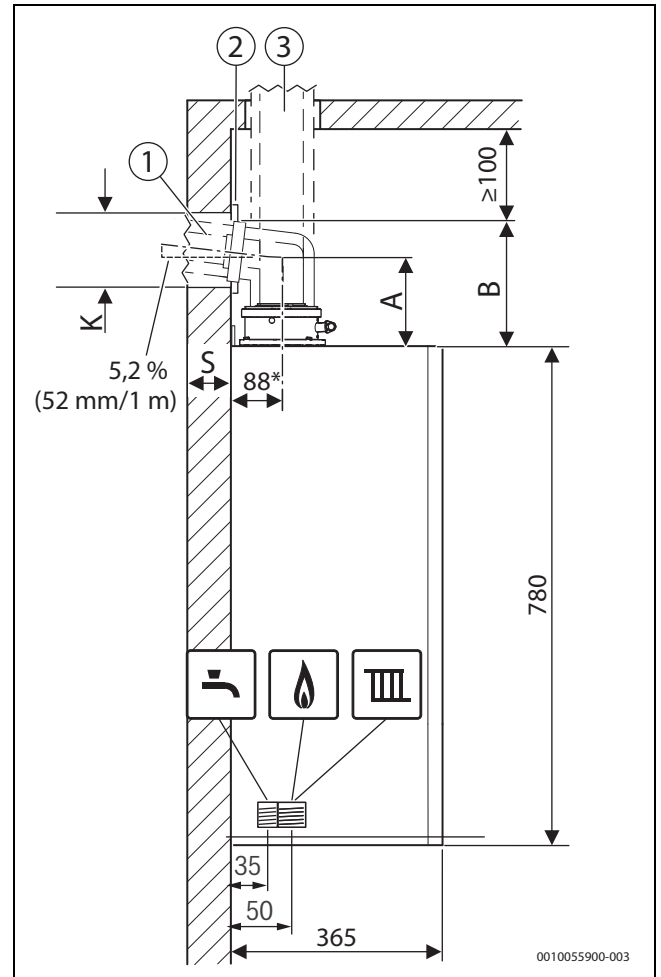
Bild 2 Seitenansicht (mm)
