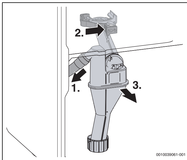
Bild 85 Kondensatsiphon ausbauen
