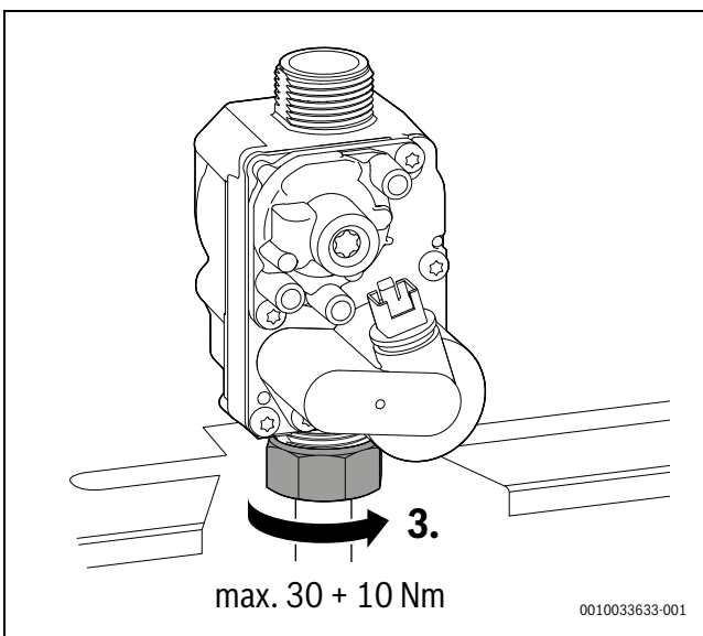
Bild 81 Anzugsdrehmoment beachten
