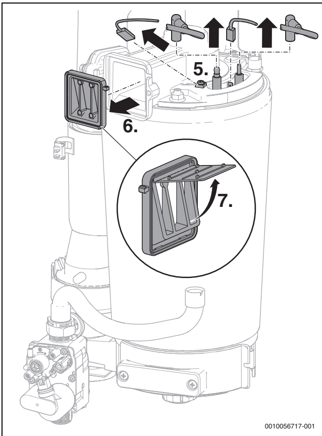
Bild 59 Kabel abziehen
