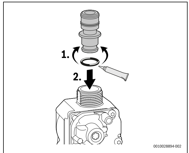
Bild 82 Gasdrossel einsetzen
