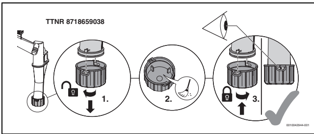
Bild 86 Schmutzfänger reinigen
