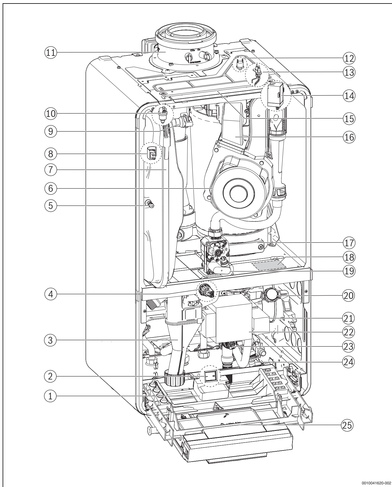
Bild 6 Produktübersicht
