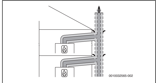
Bild 25 Mehrfachbelegung nach C (12)3x mit konzentrischer Luft-Abgas-Führung im Aufstellraum
