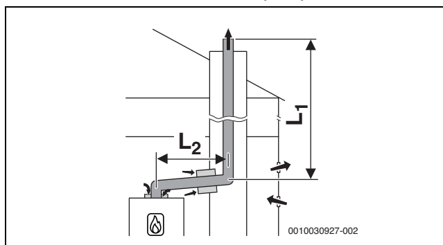
Bild 22 Starre Abgasführung im Schacht nach B 23p /B 53p mit raumluftabhängiger Luftzufuhr am Gerät und konzentrischem Verbindungsstück zwischen Aufstellraum und Schacht
