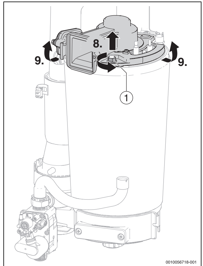
Bild 60 Brennerdeckel mit Gebläse und Mischeinrichtung abnehmen
