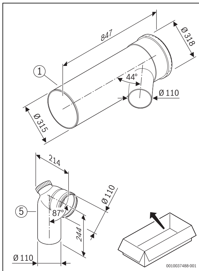
2 Ø 315: 7736701949
