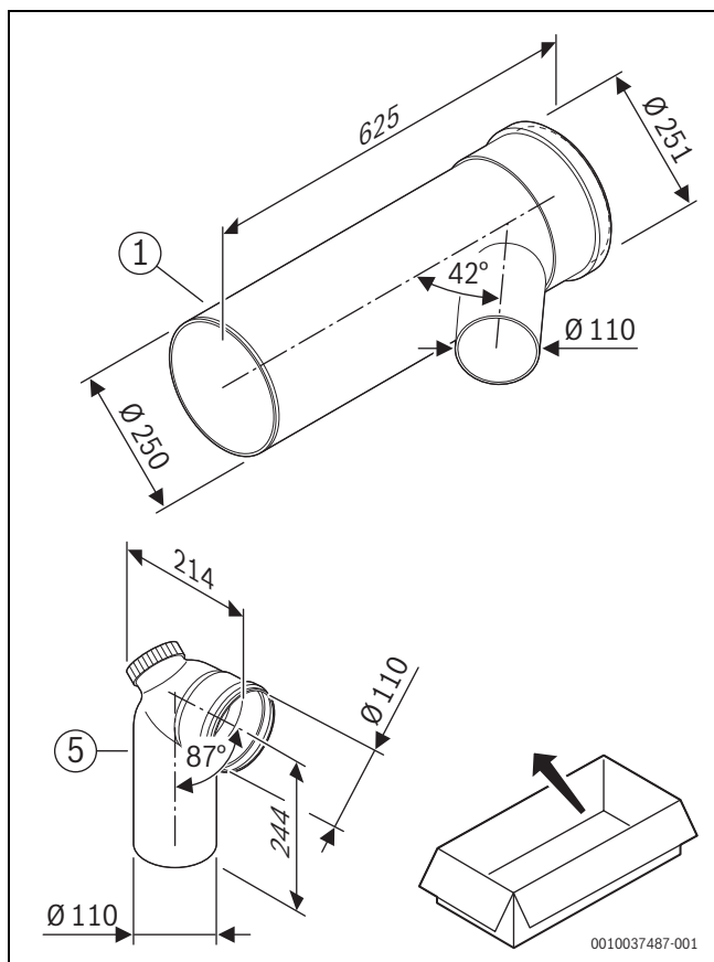
1 Ø 250: 7736701948
