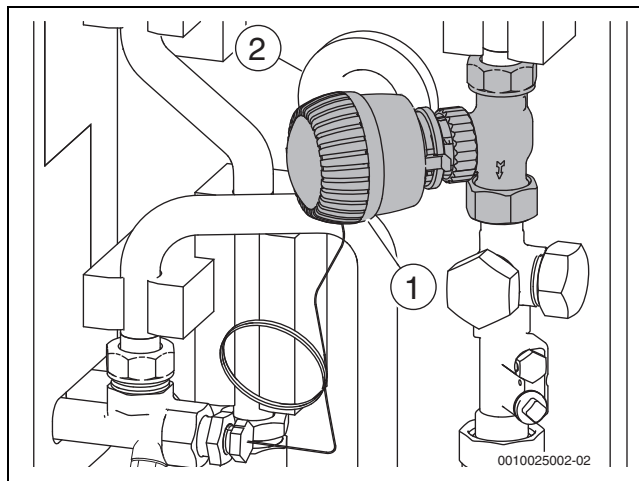
Bild 16 Warmwassertemperatur einstellen
