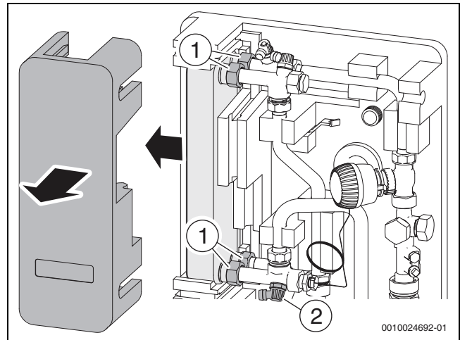
Bild 23 Wärmetauscher demonstrieren
