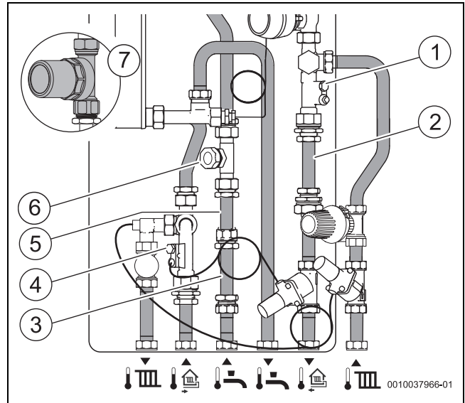
Bild 14 Adapterrohre ersetzen
