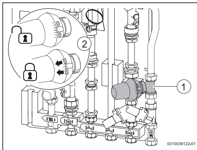
Bild 18 Rücklauftemperaturbegrenzer
