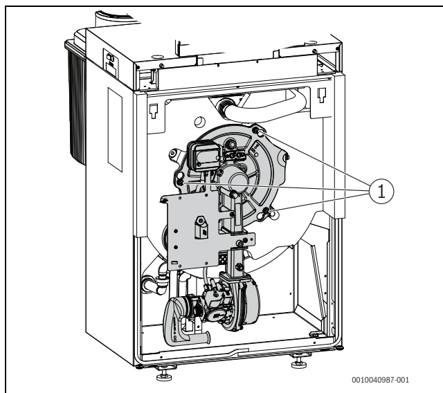
Fig. 25 Løsn fastspændingsmøtrikkerne
