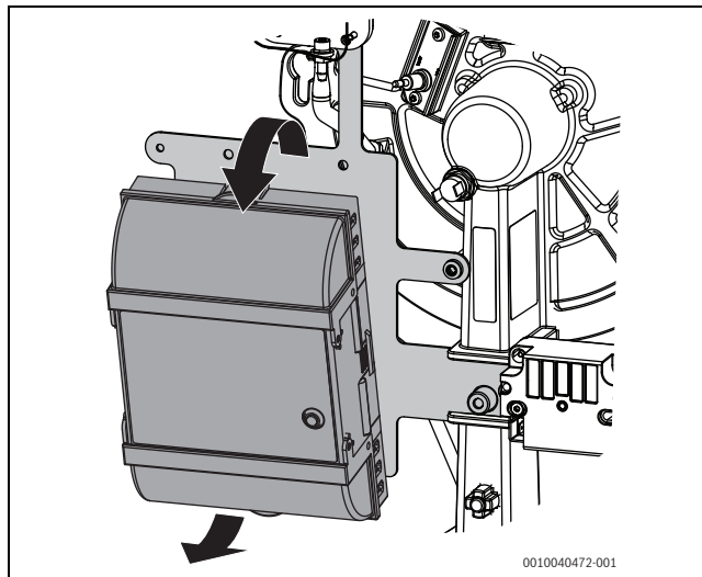
Afb. 68 Branderautomaat losmaken
