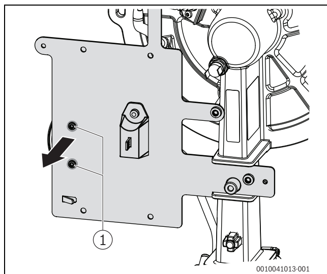
Fig. 60 Smontare il pressostato basso carico
