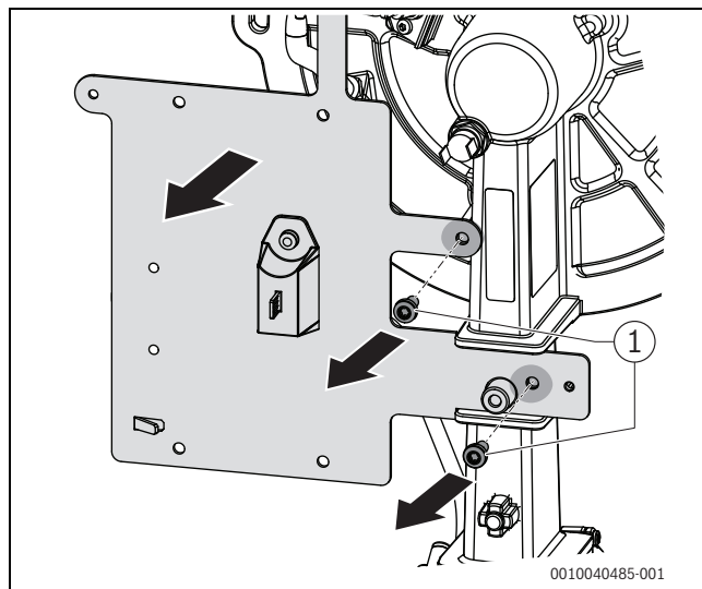
Fig. 61 Smontare il lamierino di supporto
