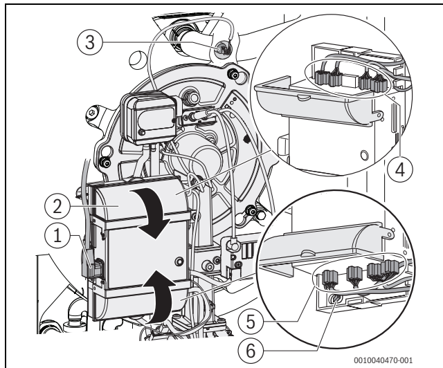
Afb. 67 Steekverbindingen losmaken
