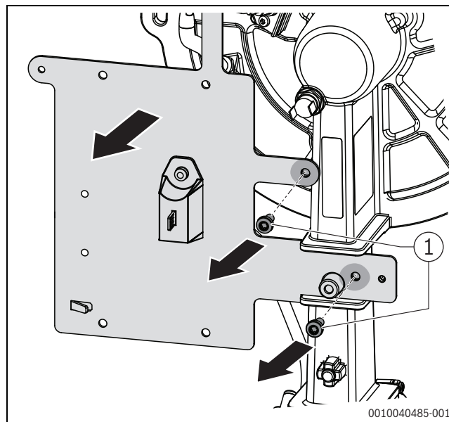
Bild 13 Halteblech demontieren
