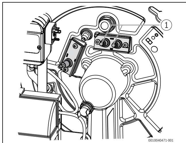
Fig. 21 Tændelegtrode
