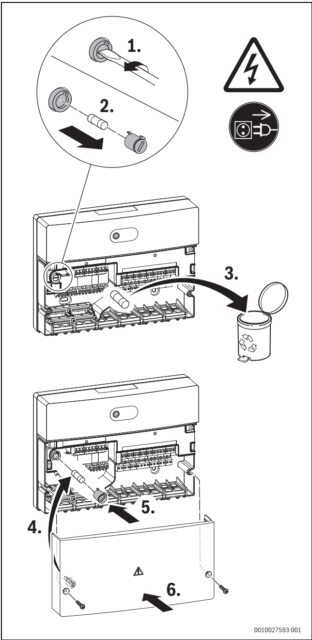
Bild 26 Sicherung tauschen
