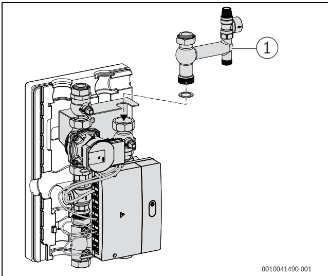
Bild 6 Sicherheitsventil montieren
