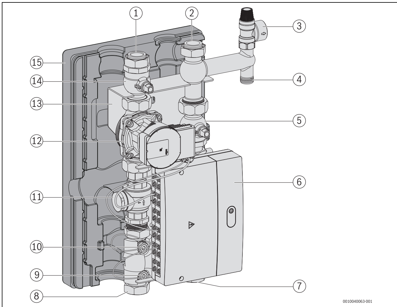
Bild 4 Produktübersicht (Dargestellt: Anschluss-Set HW)
