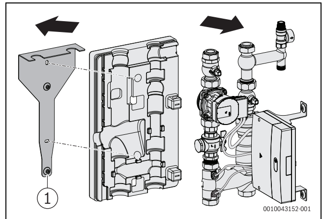
Bild 8 Wandhalterung entnehmen
