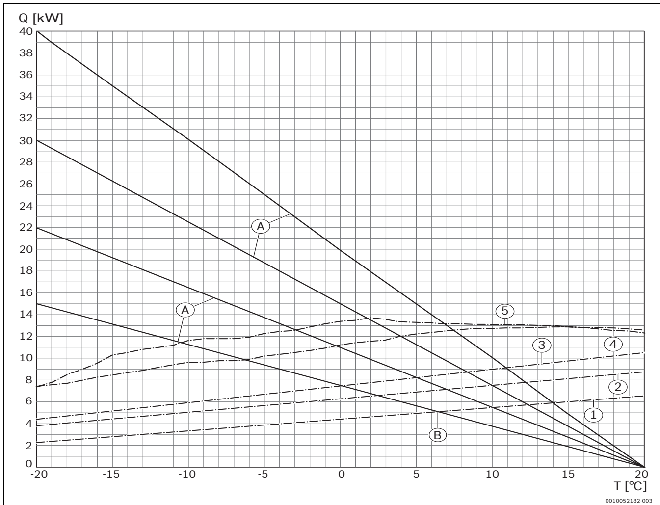
Bild 31 Diagramm zu Tab. 16; Zur Bestimmung der Bivalenzpunkte bei 45 °C Vorlauftemperatur
