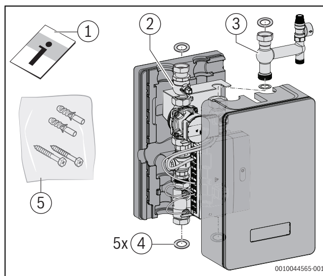
Bild 3 Lieferumfang HW-Set HYC25
