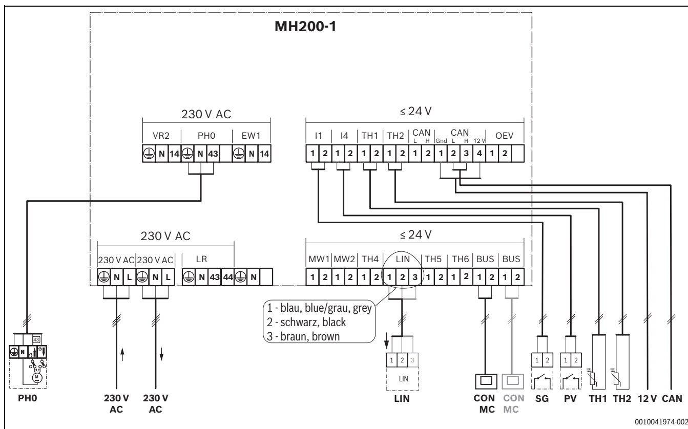
Bild 23 Überblick Anschlussklemmenbelegung
