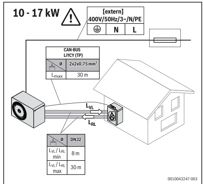
Bild 13 Anforderungen an Leitungslängen 10-17 kW
