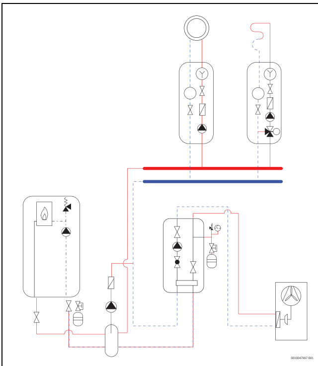
Bild 8 Hydraulisches Schema für Systeme mit mehreren Heizkreisen
