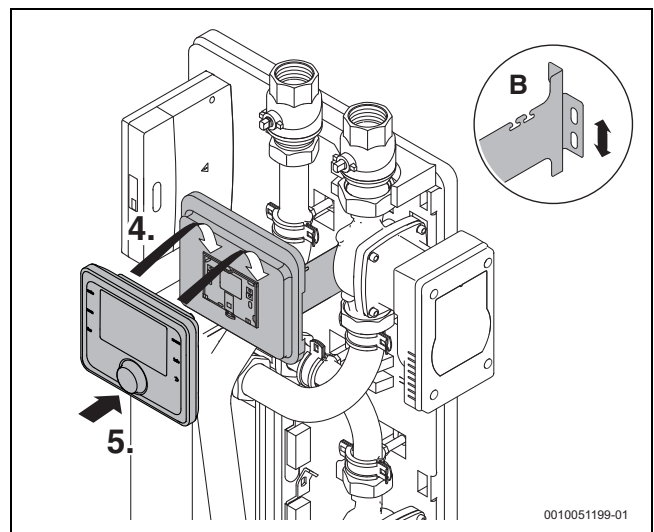
Bild 29 Bedieneinheit montieren
