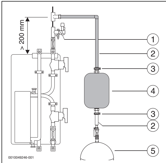
Bild 21 Vorschaltgefäß anschließen
