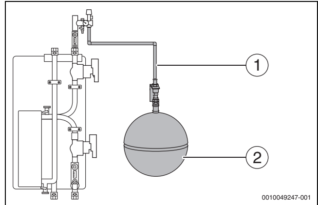
Bild 22 Ausdehnungsgefäß montieren
