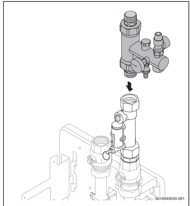
Bild 20 Sicherheitsgruppe montieren
