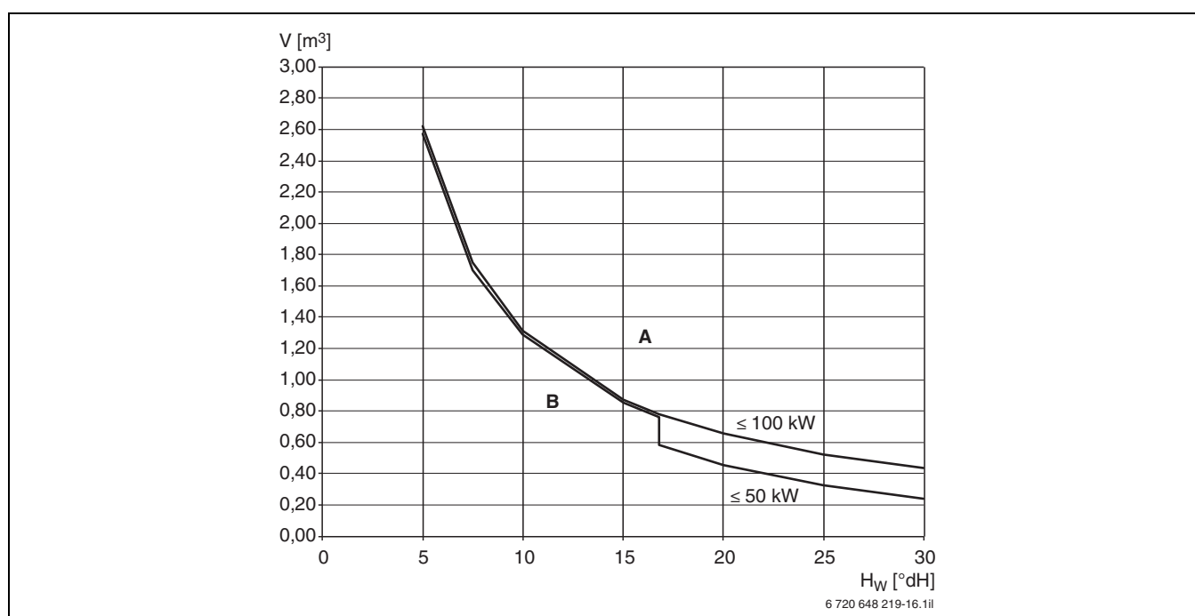
Bild 9 Grenzen zur Wasserbehandlung bei 1-Kessel-Anlagen ≤ 50 kW und ≤ 100 kW
