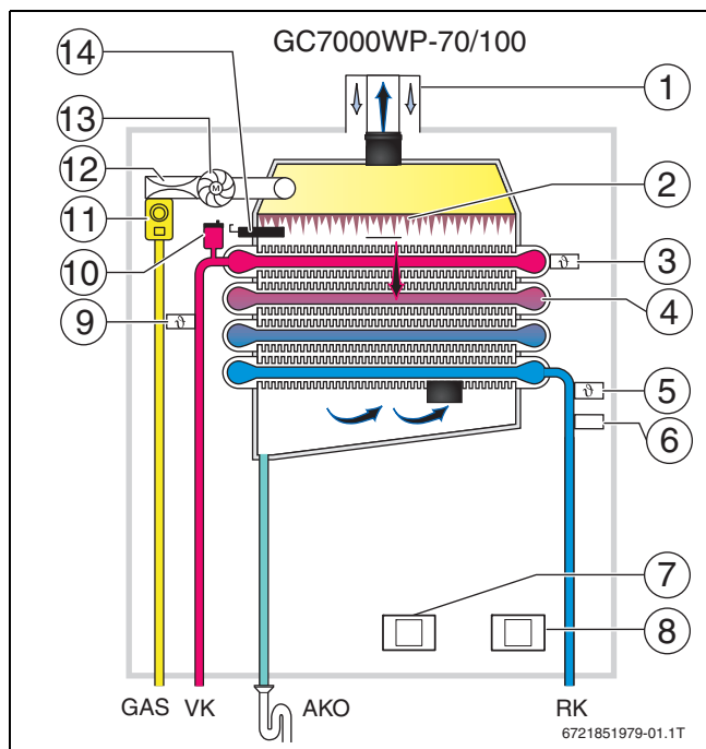
Bild 3 Funktionsschema Condens 7000 WP
