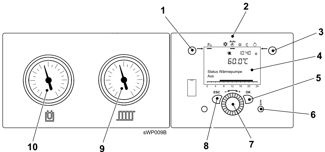
Abb. 2: Bedienelemente
