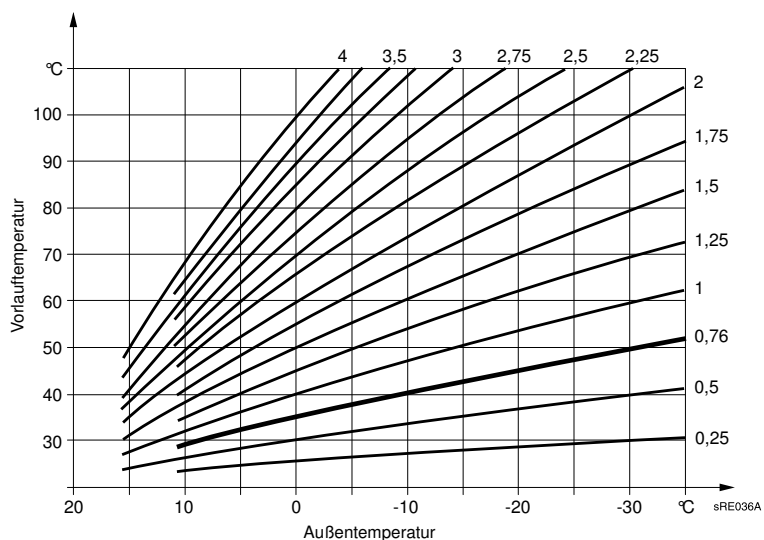
Abb. 5: Heizkennlinie
