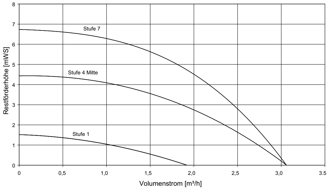
Abb. 9: Restförderhöhe Kondensatorseite BSW 13 - 15
