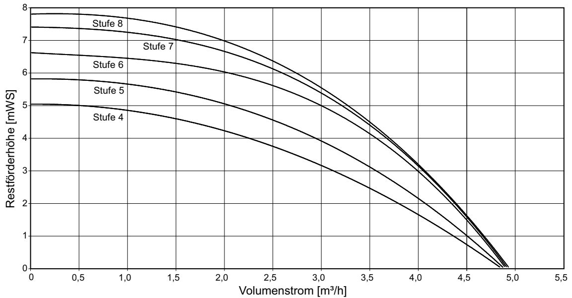
Abb. 10: Restförderhöhe Verdampferseite BSW 13
