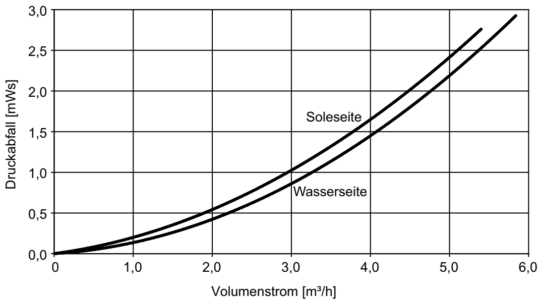
Abb. 12: Druckabfall BSW 21
