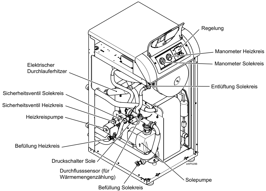
Abb. 14: Geräteansicht BSW 6-15
