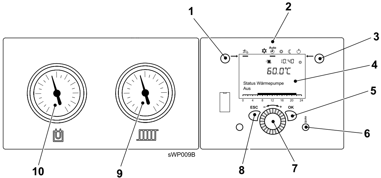
Abb. 16: Bedienelemente
