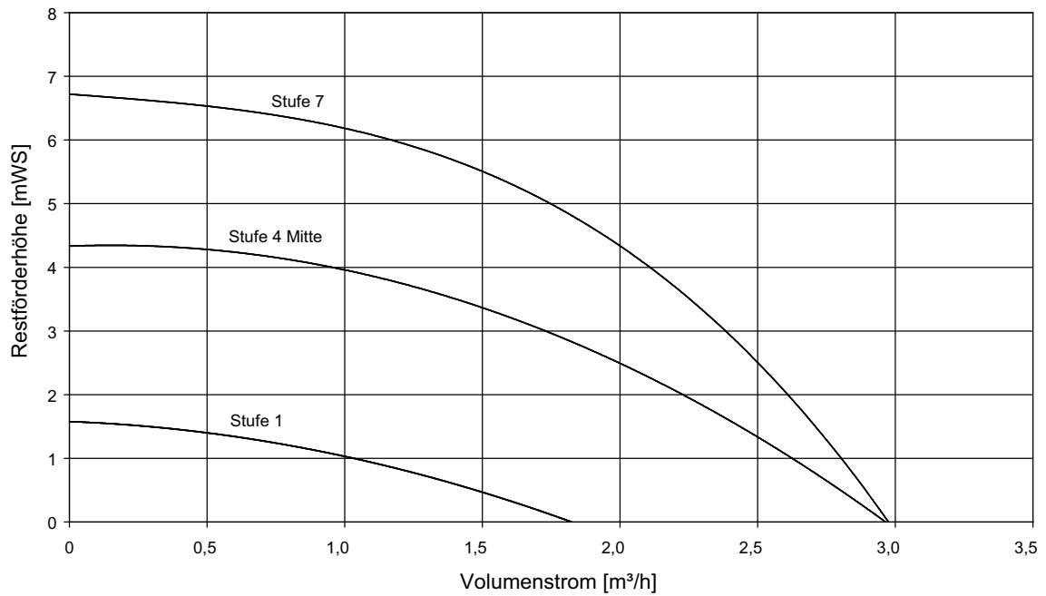
Abb. 7: Restförderhöhe Kondensatorseite BSW 10
