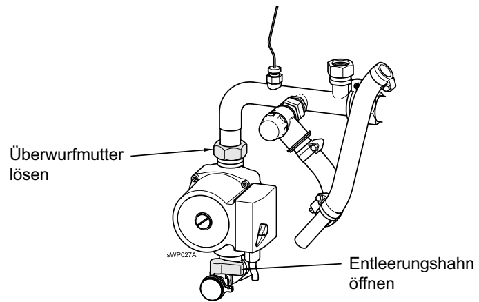
Abb. 42: Heizkreispumpe ausbauen
