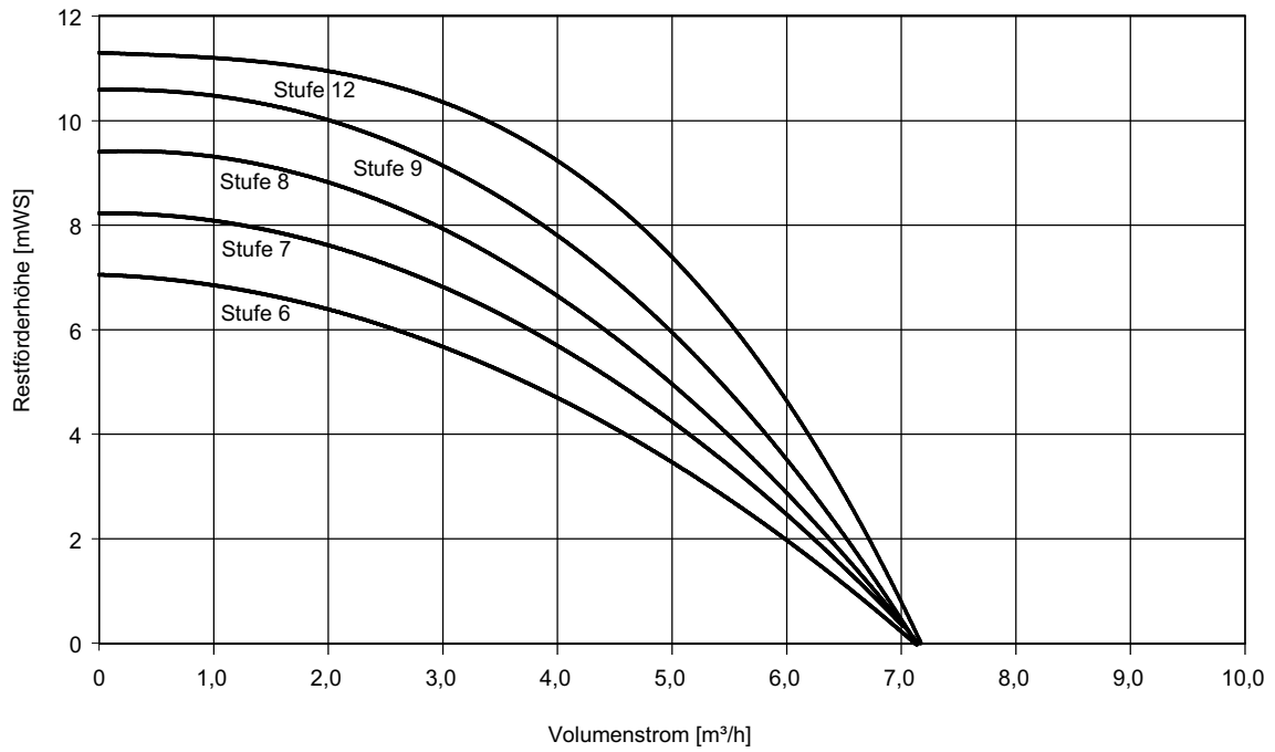
Abb. 11: Restförderhöhe Verdampferseite BSW 15
