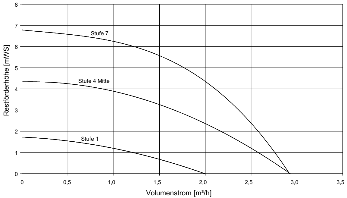
Abb. 5: Restförderhöhe Kondensatorseite BSW 8
