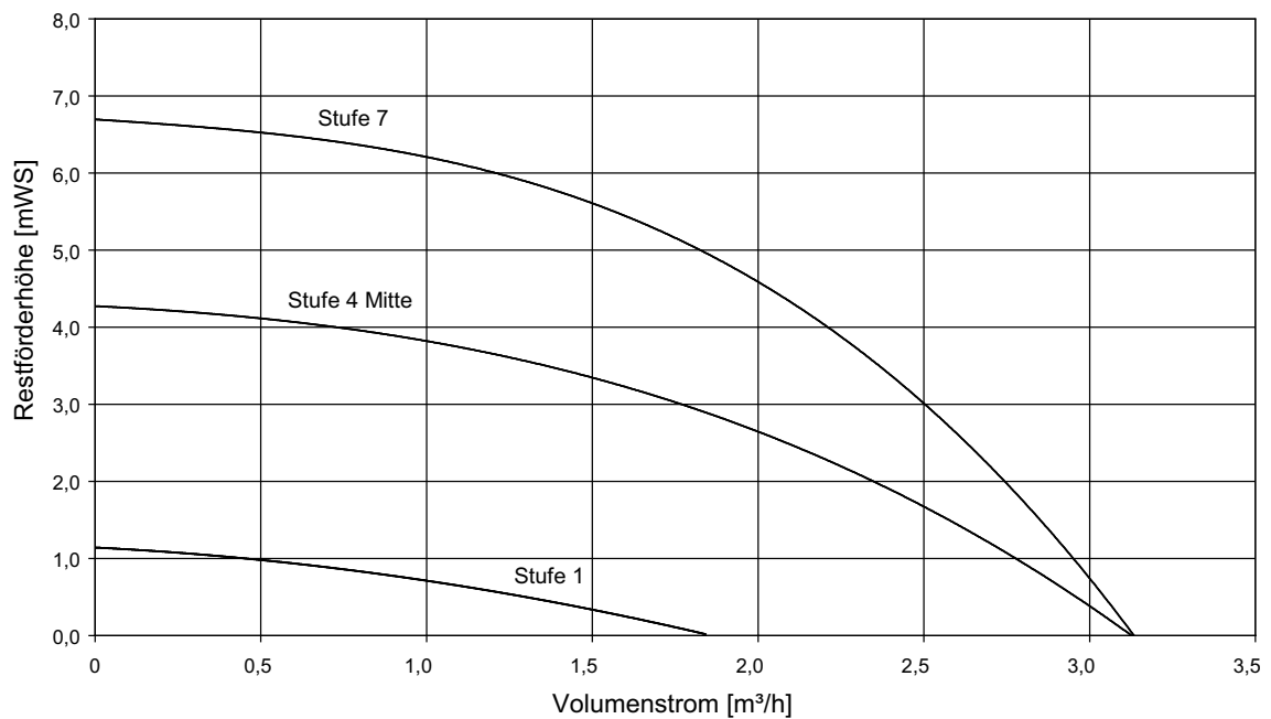
Abb. 4: Restförderhöhe Verdampferseite BSW 6 / 7
