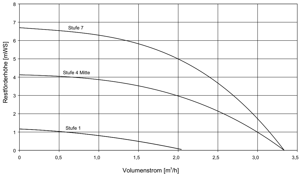
Abb. 6: Restförderhöhe Verdampferseite BSW 8
