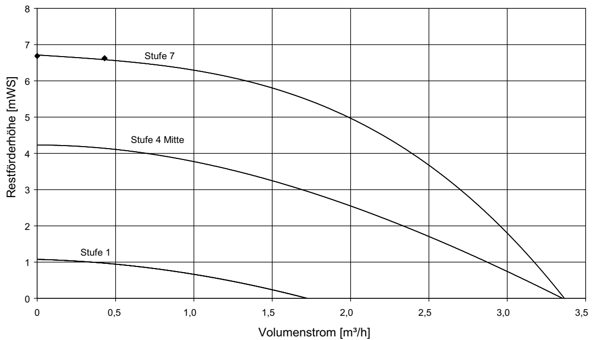
Abb. 8: Restförderhöhe Verdampferseite BSW 10
