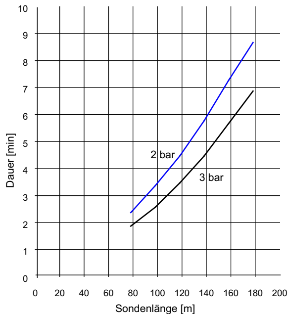
Abb. 26: Mindestspüldauer (Sondendurchmesser 32 mm)
