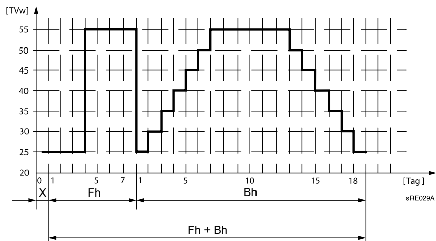
Abb. 34: Temperaturprofil bei der Estrich-Austrocknungsfunktion
