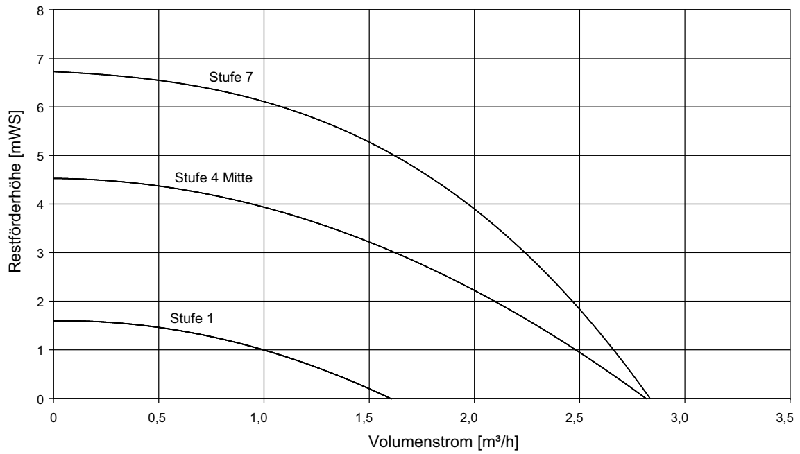
Abb. 3: Restförderhöhe Kondensatorseite BSW 6 / 7
