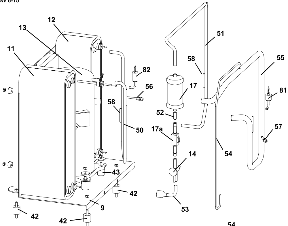
Abb. 46: Kältekreis
