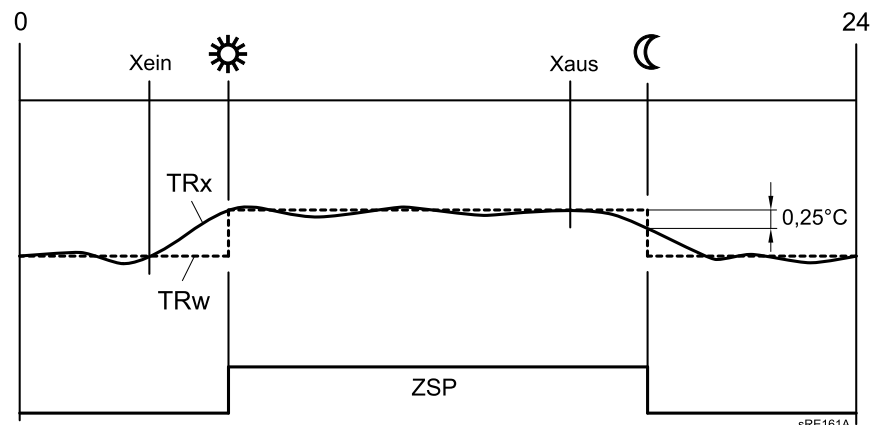
Abb. 32: Einschalt- und Ausschaltoptimierung
