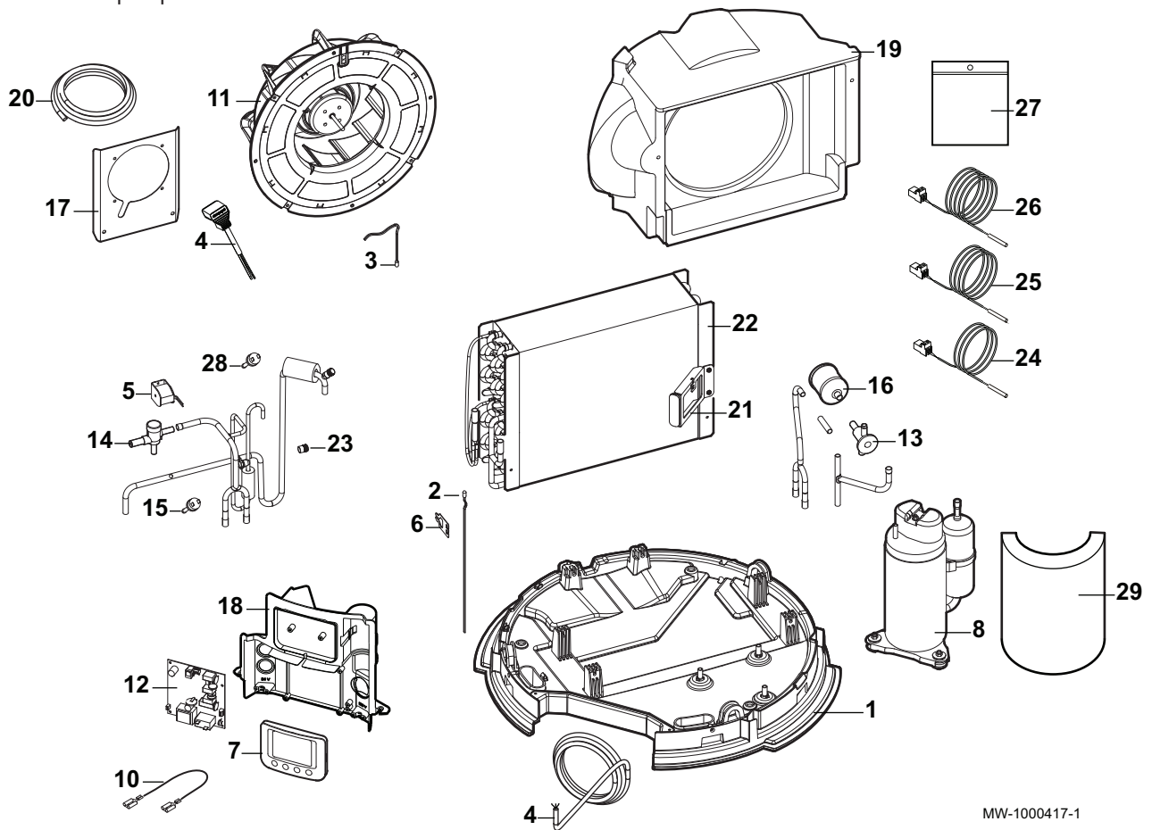
Abb.56 Wärmepumpe
