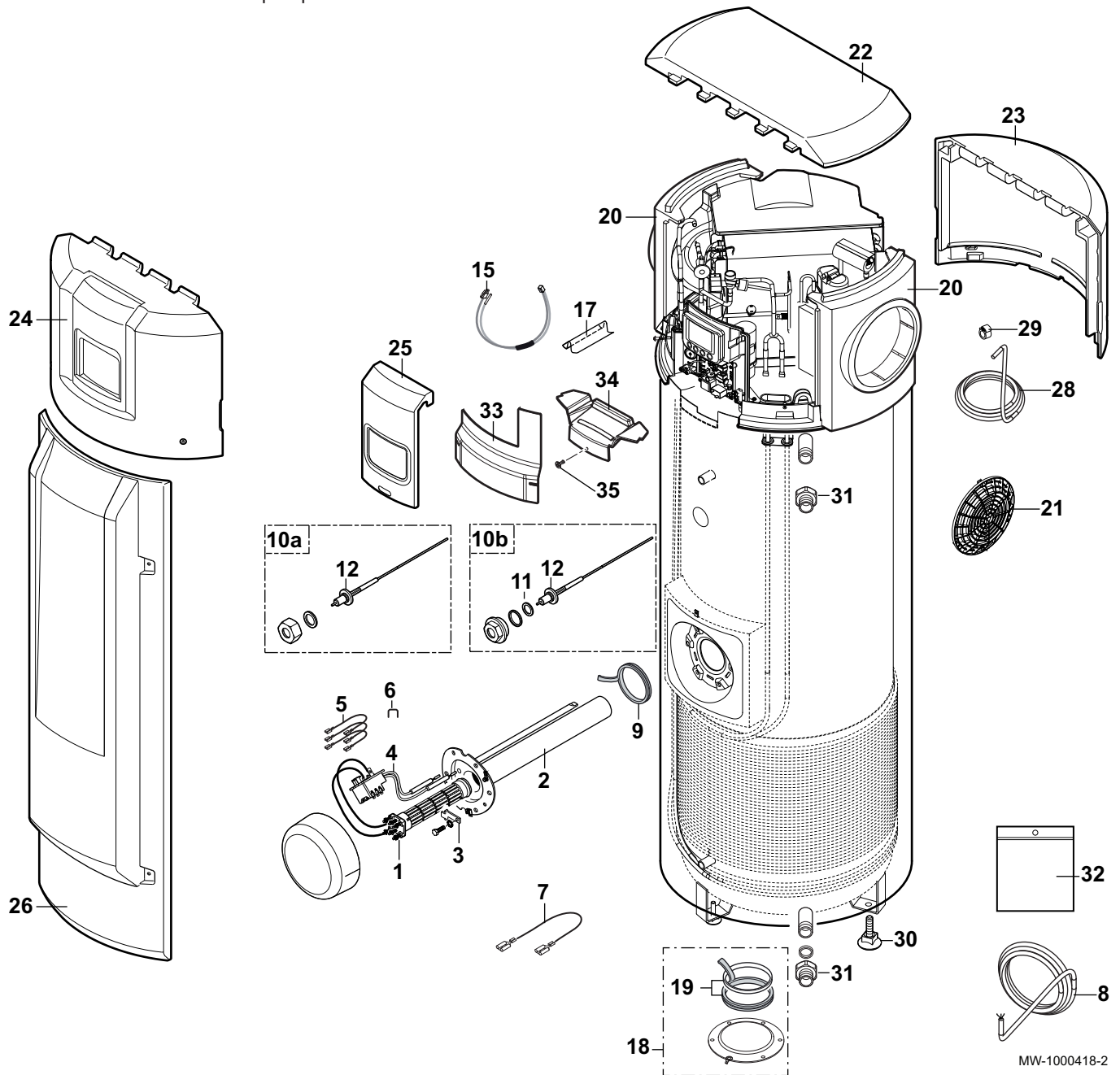
Abb.57 Trinkwasser-Wärmepumpe
