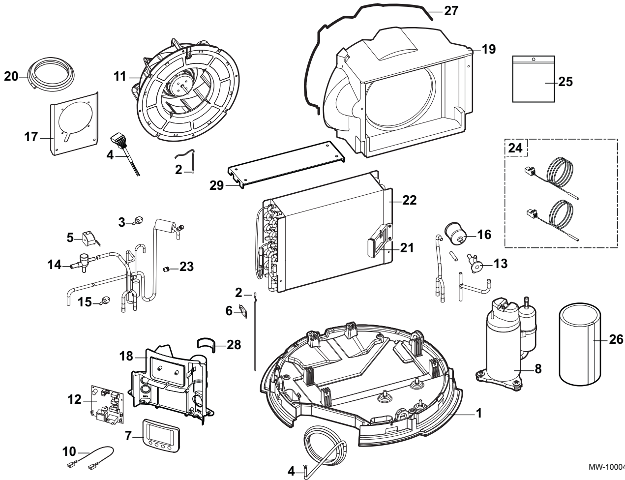
Abb.58 Wärmepumpe
