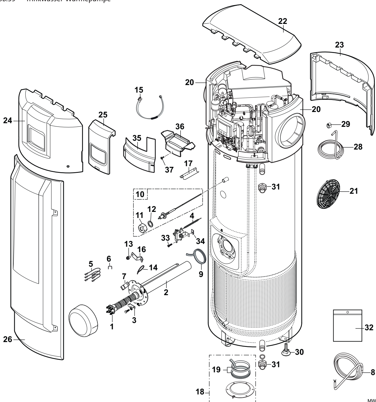
Abb.59 Trinkwasser-Wärmepumpe
