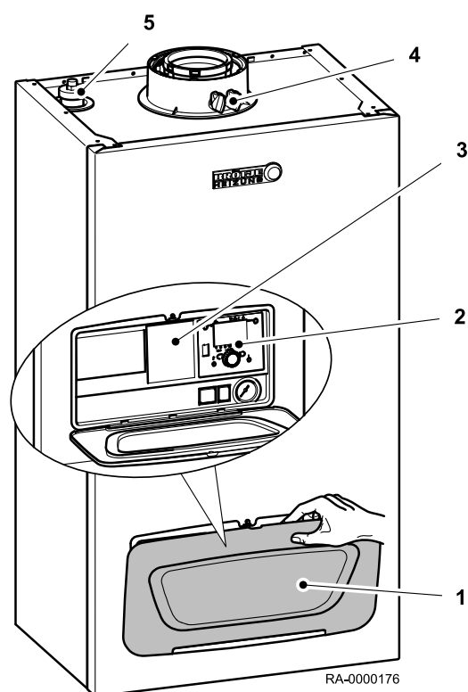
Abb.1 Übersichtszeichnung WGB-C/-U
