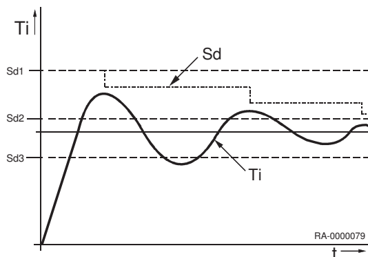
Abb.36 Schaltdifferenz
