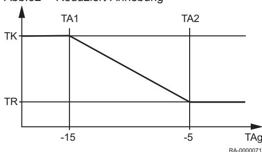
Abb.32 Reduziert-Anhebung
