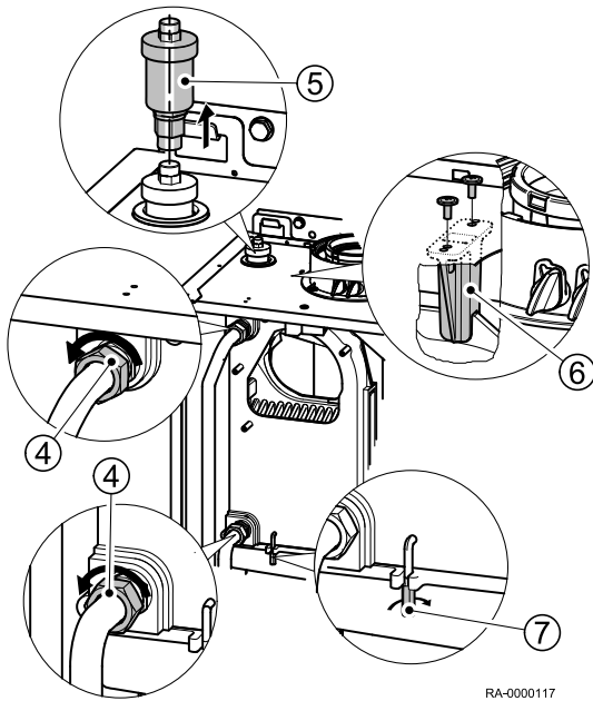
Abb.46 Wärmetauscher ausbauen
