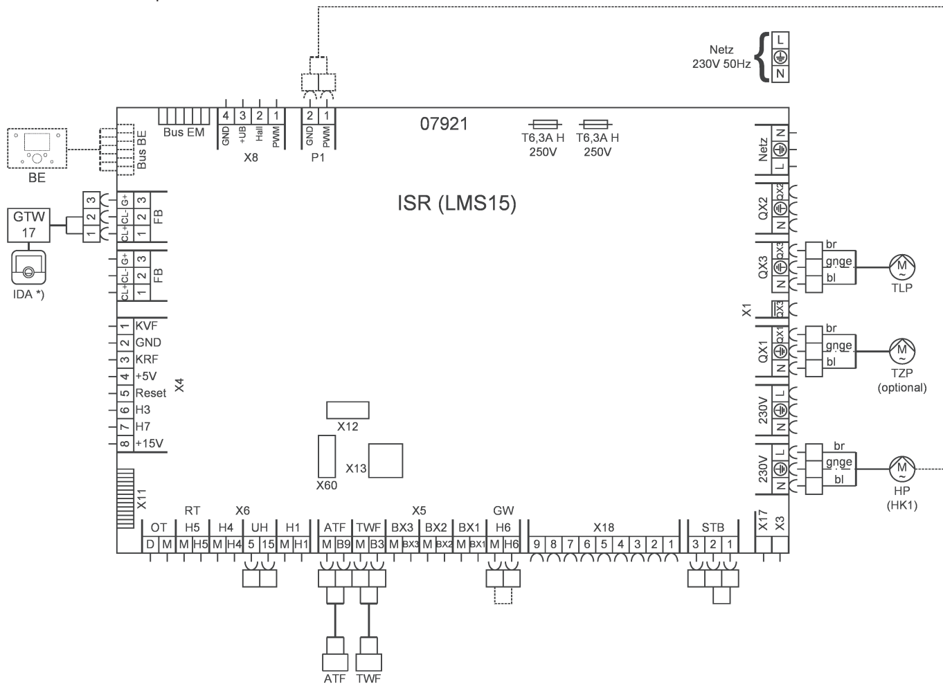
Abb.13 Anschlussplan
