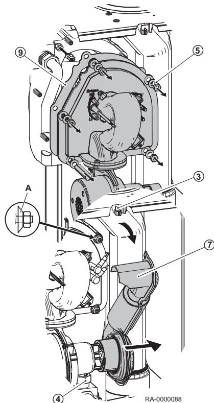
Abb.45 Gasbrenner ausbauen
