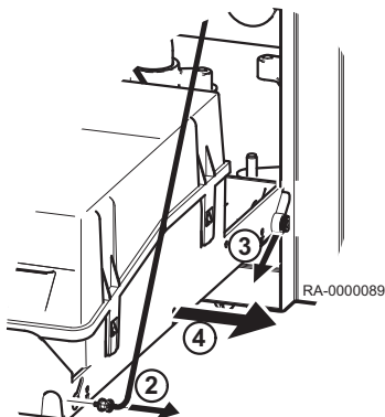
Abb.42 Kesselschaltfeld aushaken
