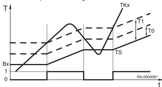
Abb.38 Speicherladung
