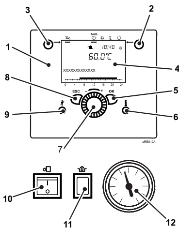
Abb.8 Bedienelemente
