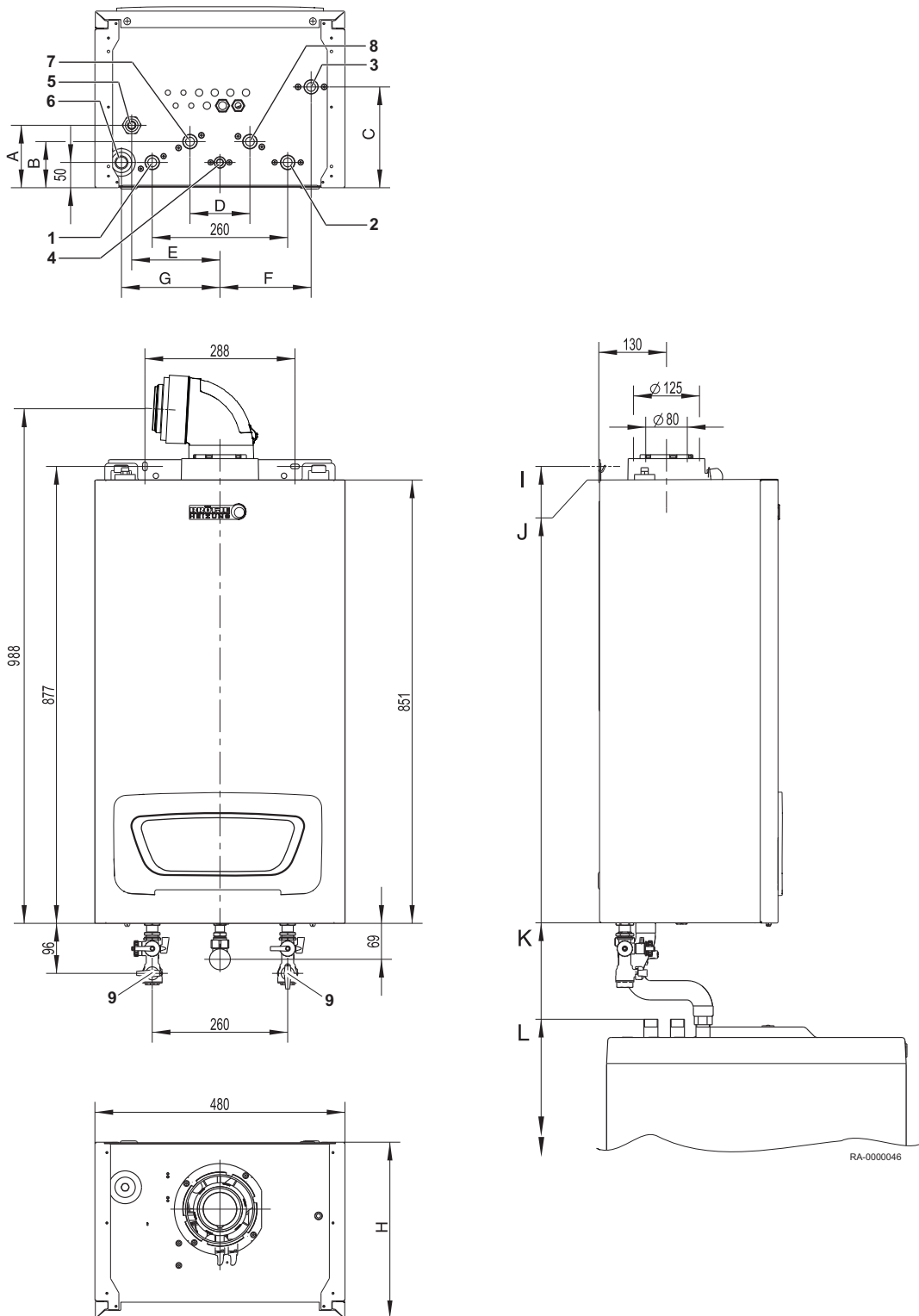
Abb.4 Abmessungen und Anschlüsse WGB EVO
