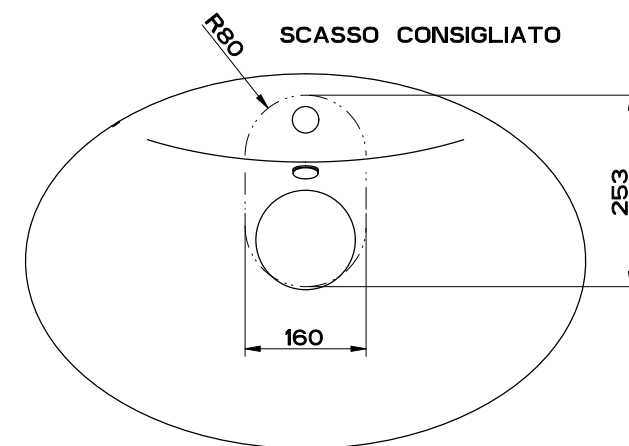
SCASSO CONSIGLIATO
