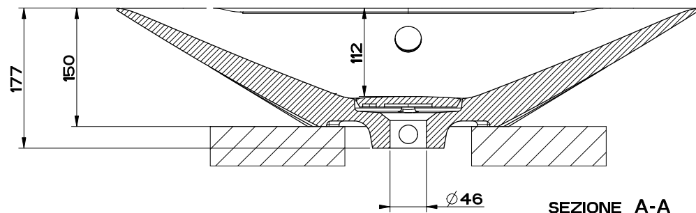
SEZIONE A-A
