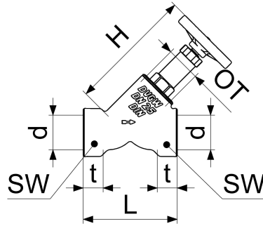
Masszeichnung
