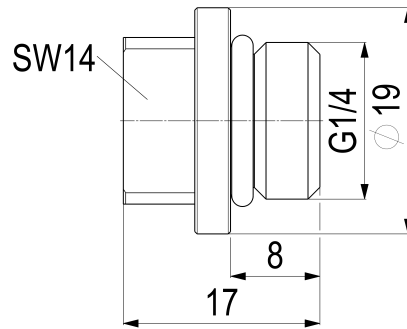
Masszeichnung
